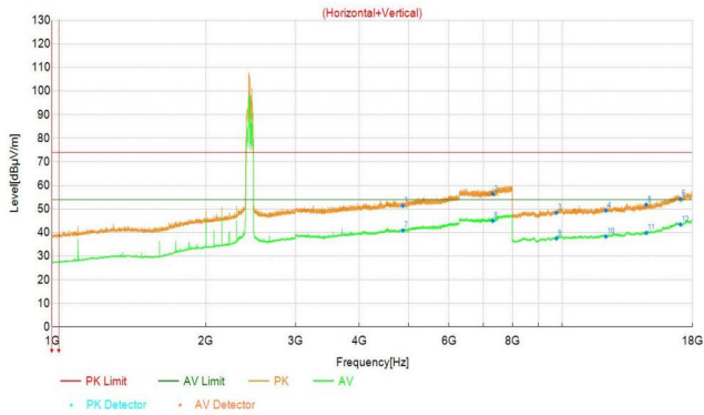
11AX_20M_2412
