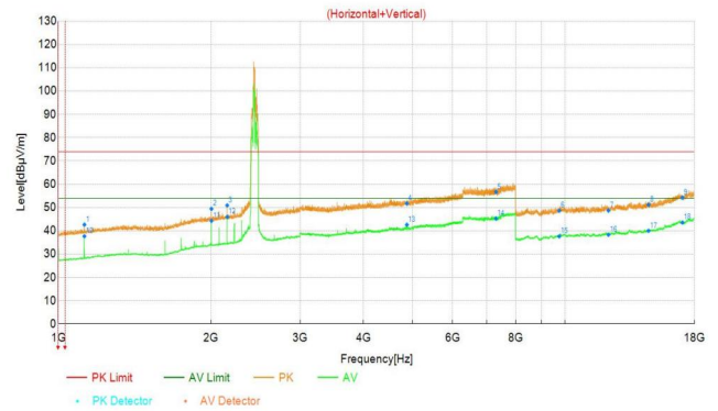
11N_40M_2422
