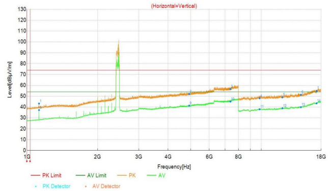
11AX_20M_2437
