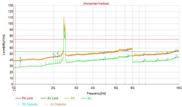
11AX_20M_2462
