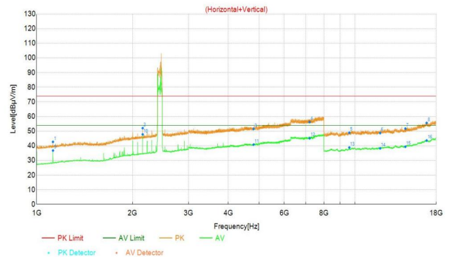
BLE_2M_2480
