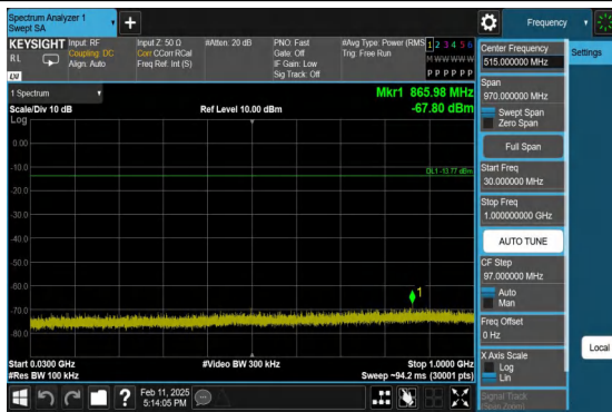
BLE_500K-Ant1-2440-30~1000-PASS
