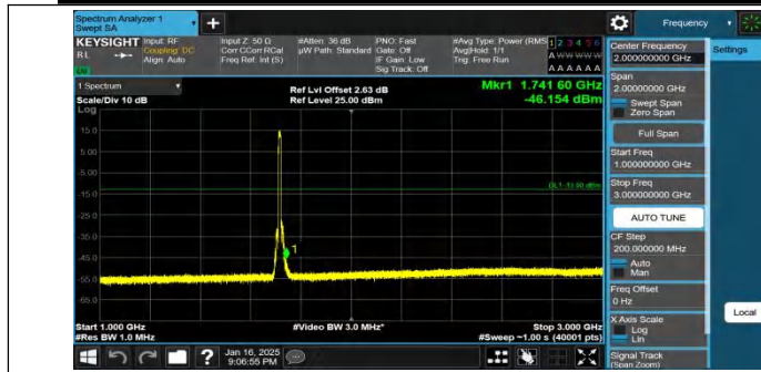
Band4-10MHz-QPSK-20000-50RB#0-1000~3000-PASS
