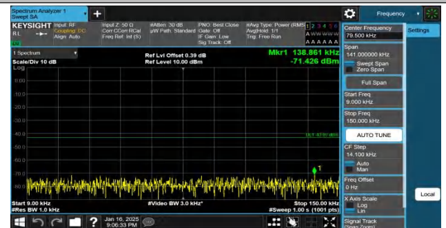
Band4-10MHz-QPSK-20000-50RB#0-0.009~0.15-PASS
