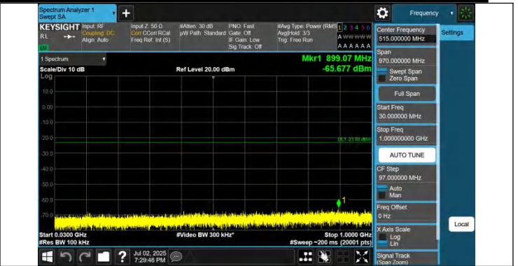
42-42-20MHz-20MHz-QPSK-QPSK-42491-42689-1RB#99-0RB# 0-30~1000MHz-PASS
