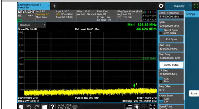
42-42-20MHz-20MHz-QPSK-QPSK-42792-42990-1RB#99-0RB# 0-30~1000MHz-PASS
