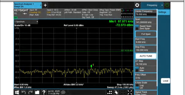
42-42-20MHz-20MHz-QPSK-QPSK-42491-42689-1RB#99-0RB# 0-0.009~0.15MHz-PASS
