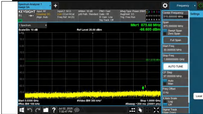
42-42-20MHz-10MHz-QPSK-QPSK-42891-43035-1RB#99-0RB# 0-30~1000MHz-PASS
