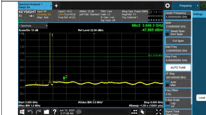
42-42-20MHz-10MHz-QPSK-QPSK-42891-43035-1RB#99-0RB# 0-3000~6000MHz-PASS
