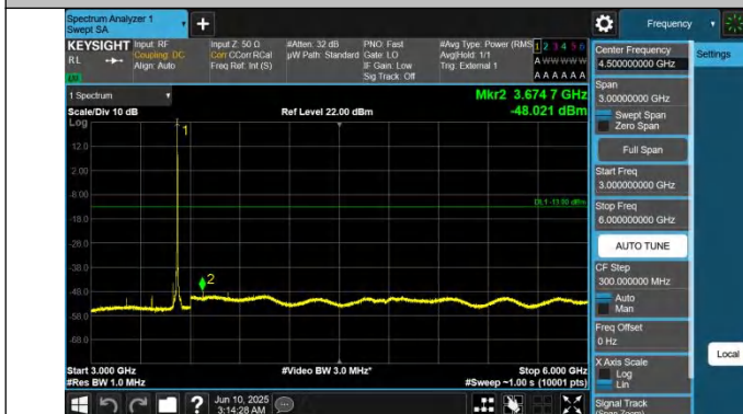
42-42-20MHz-10MHz-QPSK-QPSK-42891-43035-1RB#0-0RB#0- 3000~6000MHz-PASS
