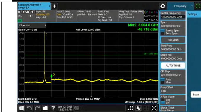
42-42-20MHz-20MHz-QPSK-QPSK-42190-42388-1RB#0-0RB#0-3000~6000MHz-PASS
