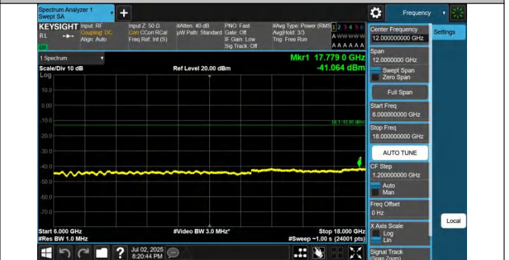
42-42-20MHz-10MHz-QPSK-QPSK-42891-43035-1RB#99-0RB# 0-6000~18000MHz-PASS
