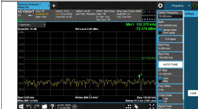
42-42-20MHz-20MHz-QPSK-QPSK-42792-42990-1RB#99-0RB# 0-0.009~0.15MHz-PASS
