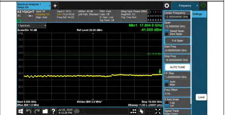
42-42-20MHz-20MHz-QPSK-QPSK-42190-42388-1RB#99-0RB# 0-6000~18000MHz-PASS
