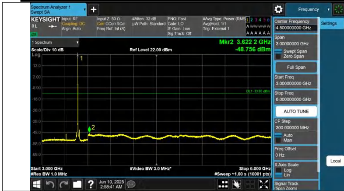
42-42-20MHz-10MHz-QPSK-QPSK-42190-42334-1RB#99-0RB# 0-3000~6000MHz-PASS
