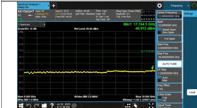
42-42-20MHz-5MHz-QPSK-QPSK-42940-43057-1RB#99-0RB#0- 6000~18000MHz-PASS
