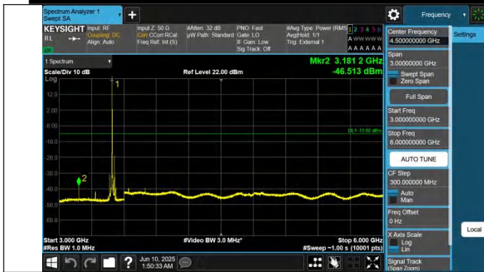
42-42-20MHz-5MHz-QPSK-QPSK-42565-42682-1RB#0-0RB#0-3 000~6000MHz-PASS
