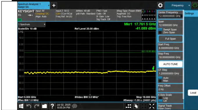
42-42-5MHz-20MHz-QPSK-QPSK-42873-42990-1RB#0-1RB#99- 6000~18000MHz-PASS
