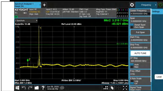
42-42-5MHz-20MHz-QPSK-QPSK-42873-42990-1RB#0-0RB#0-3 000~6000MHz-PASS
