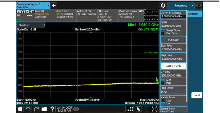
42-42-10MHz-20MHz-QPSK-QPSK-42145-42289-1RB#0-1RB#9 9-1000~3000MHz-PASS
