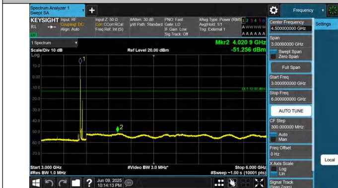
42-42-10MHz-20MHz-QPSK-QPSK-42846-42990-1RB#0-1RB#99-9-3000~6000MHz-PASS
