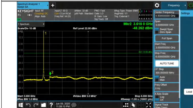
42-42-15MHz-20MHz-QPSK-QPSK-42168-42339-1RB#74-0RB# 0-3000~6000MHz-PASS
