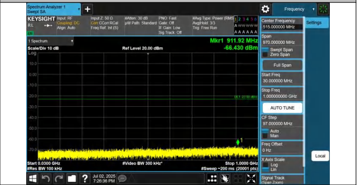
42-42-10MHz-20MHz-QPSK-QPSK-42145-42289-1RB#0-0RB#0-30~1000MHz-PASS
