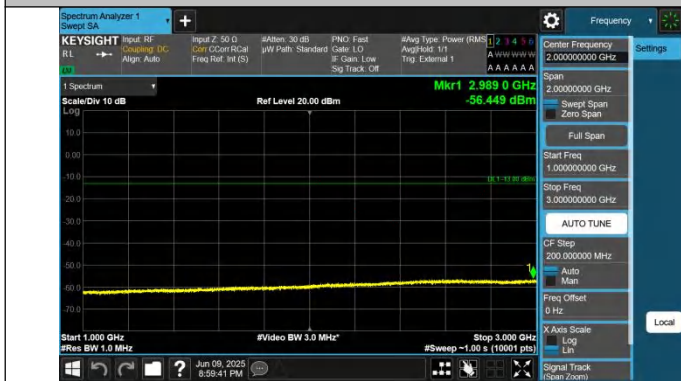
42-42-5MHz-20MHz-QPSK-QPSK-42873-42990-1RB#0-1RB#99- 1000~3000MHz-PASS
