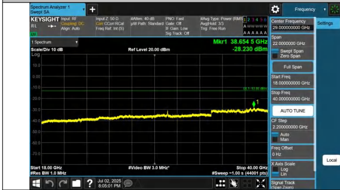
42-42-5MHz-20MHz-QPSK-QPSK-42873-42990-1RB#0-0RB#0-1 8000~40000MHz-PASS
