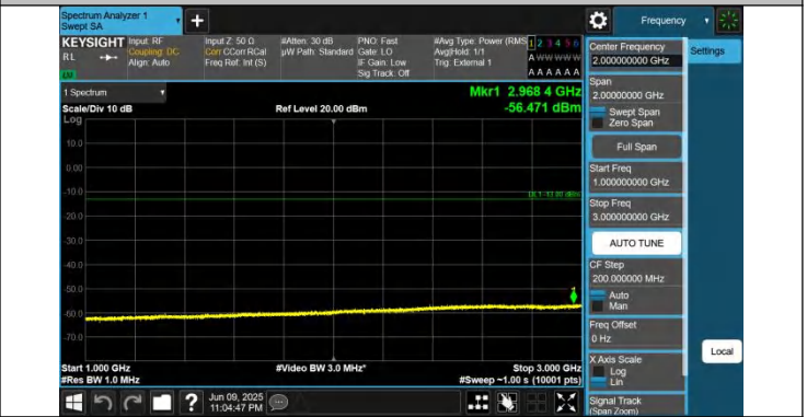
42-42-15MHz-20MHz-QPSK-QPSK-42168-42339-1RB#0-0RB#0- 1000~3000MHz-PASS
