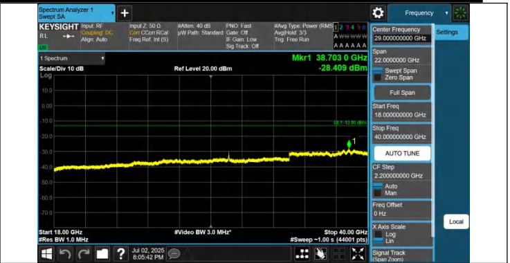
42-42-5MHz-20MHz-QPSK-QPSK-42873-42990-1RB#0-1RB#99- 18000~40000MHz-PASS
