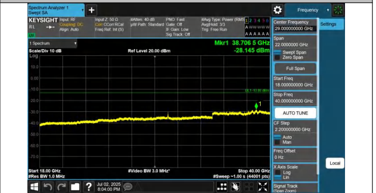
42-42-5MHz-20MHz-QPSK-QPSK-42498-42615-1RB#0-0RB#0-1 8000~40000MHz-PASS
