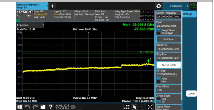
42-42-5MHz-20MHz-QPSK-QPSK-42123-42240-1RB#0-1RB#99- 18000~40000MHz-PASS
