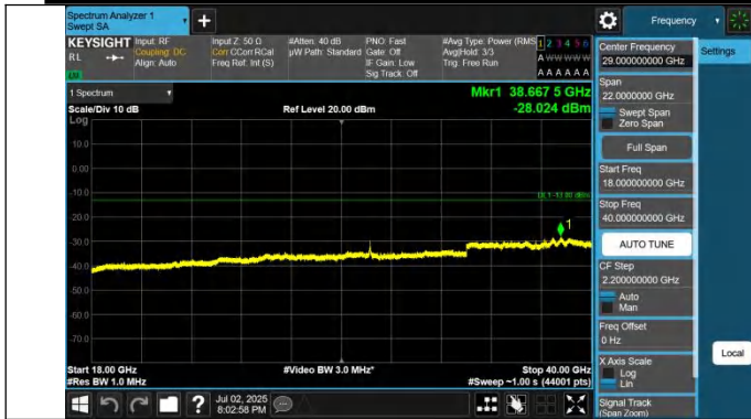
42-42-5MHz-20MHz-QPSK-QPSK-42123-42240-1RB#0-0RB#0-1 8000~40000MHz-PASS
