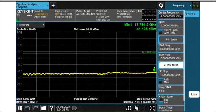
42-42-5MHz-20MHz-QPSK-QPSK-42498-42615-1RB#0-1RB#99- 6000~18000MHz-PASS
