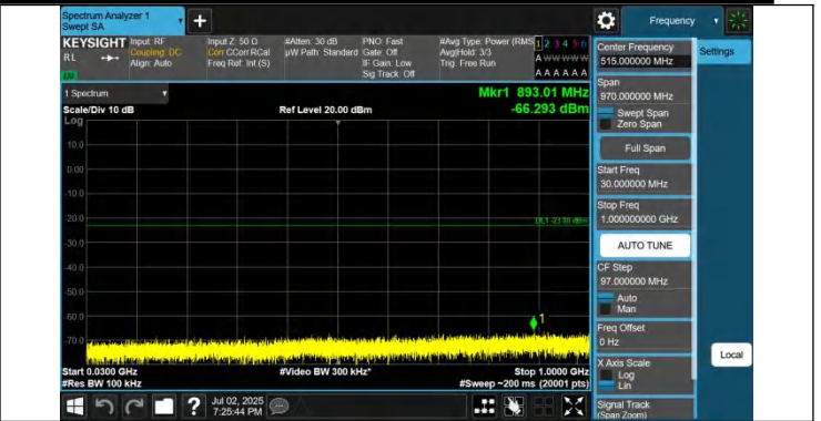
42-42-5MHz-20MHz-QPSK-QPSK-42498-42615-1RB#0-0RB#0-3 0~1000MHz-PASS
