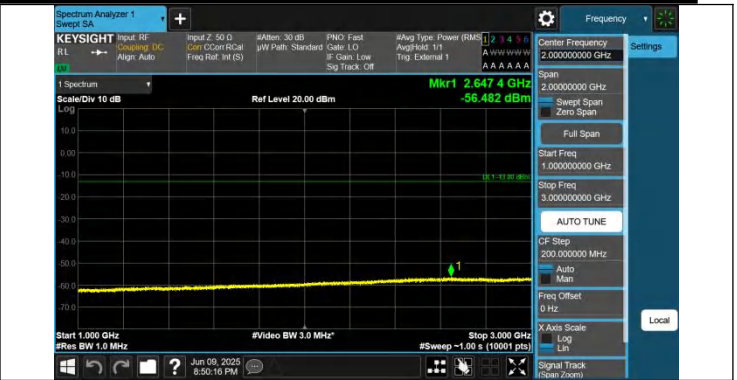
42-42-5MHz-20MHz-QPSK-QPSK-42498-42615-1RB#0-1RB#99- 1000~3000MHz-PASS
