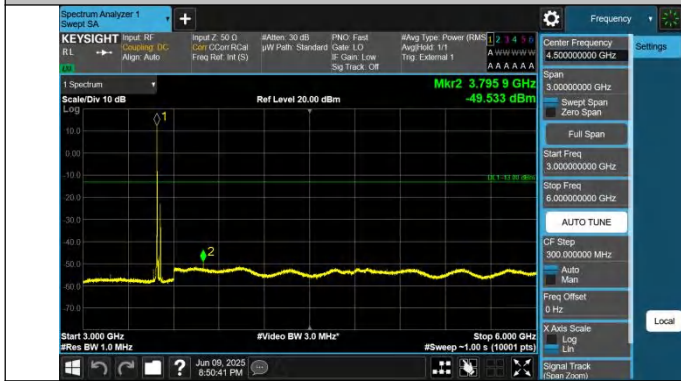
42-42-5MHz-20MHz-QPSK-QPSK-42498-42615-1RB#0-1RB#99- 3000~6000MHz-PASS
