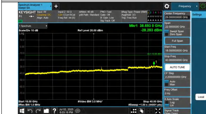
42-42-5MHz-20MHz-QPSK-QPSK-42123-42240-1RB#24-0RB#0- 18000~40000MHz-PASS
