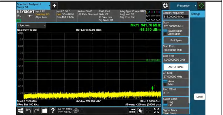
42-42-5MHz-20MHz-QPSK-QPSK-42498-42615-1RB#24-0RB#0- 30~1000MHz-PASS
