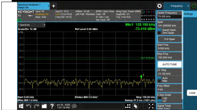
42-42-5MHz-20MHz-QPSK-QPSK-42123-42240-1RB#24-0RB#0- 0.009~0.15MHz-PASS
