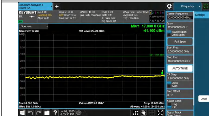
42-42-5MHz-20MHz-QPSK-QPSK-42123-42240-1RB#0-1RB#99- 6000~18000MHz-PASS
