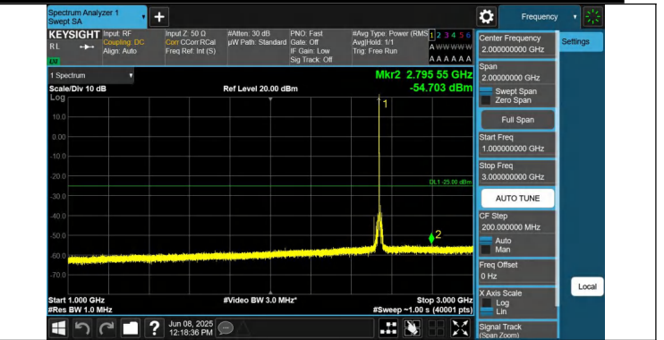
7-7-15MHz-20MHz-QPSK-QPSK-21179-21350-1RB#0-1RB#99-1 000~3000MHz-PASS
