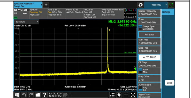
7-7-15MHz-20MHz-QPSK-QPSK-20828-20999-1RB#0-0RB#0-1000~3000MHz-PASS
