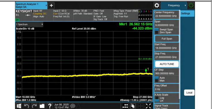
7-7-15MHz-20MHz-QPSK-QPSK-20828-20999-1RB#0-1RB#99-1 8000~27000MHz-PASS
