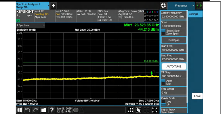
7-7-15MHz-20MHz-QPSK-QPSK-20828-20999-1RB#0-0RB#0-18 000~27000MHz-PASS
