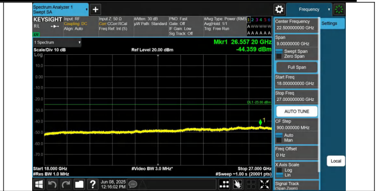
7-7-15MHz-20MHz-QPSK-QPSK-21003-21174-1RB#0-1RB#99-1 8000~27000MHz-PASS
