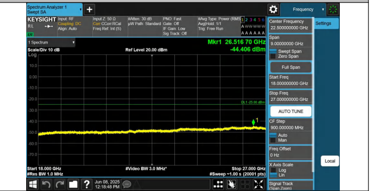
7-7-15MHz-20MHz-QPSK-QPSK-21179-21350-1RB#0-1RB#99-1 8000~27000MHz-PASS
