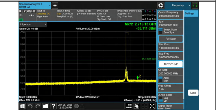
7-7-15MHz-20MHz-QPSK-QPSK-21179-21350-1RB#0-0RB#0-10 00~3000MHz-PASS
