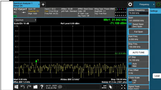
7-7-15MHz-20MHz-QPSK-QPSK-21179-21350-1RB#0-0RB#0-0. 009~0.15MHz-PASS
