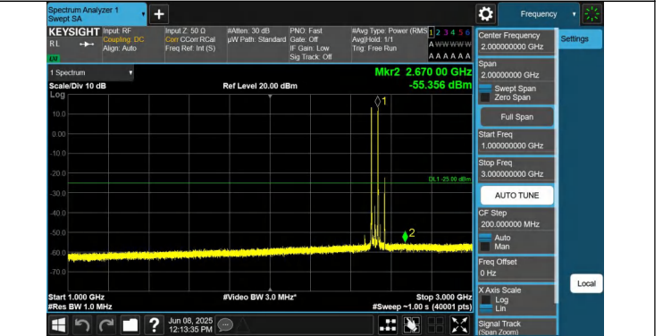
7-7-15MHz-20MHz-QPSK-QPSK-20828-20999-1RB#0-1RB#99-1 000~3000MHz-PASS
