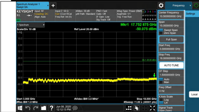
7-7-15MHz-20MHz-QPSK-QPSK-20828-20999-1RB#0-0RB#0-3 000~18000MHz-PASS
