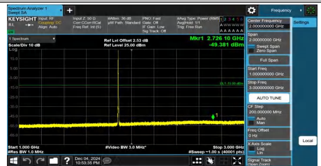
Band25-3MHz-QPSK-26365-1RB#0-1000~3000-PASS
