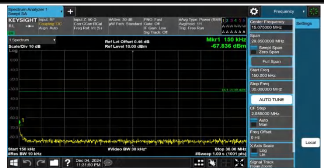
Band25-20MHz-QPSK-26365-1RB#0-0.15~30-PASS
