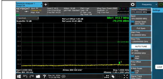
Band25-20MHz-QPSK-26365-1RB#0-30~1000-PASS
