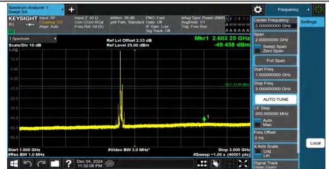
Band25-20MHz-QPSK-26365-1RB#0-1000~3000-PASS
