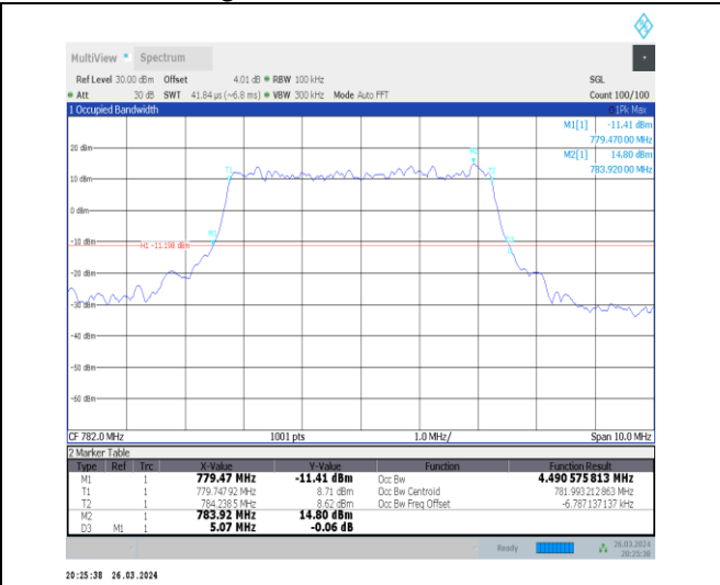
1-N13-15-5-M-6-CP-QPSK-Outer_Full-25@0-Ant1-4. 491-5.070-≤5-PASS
