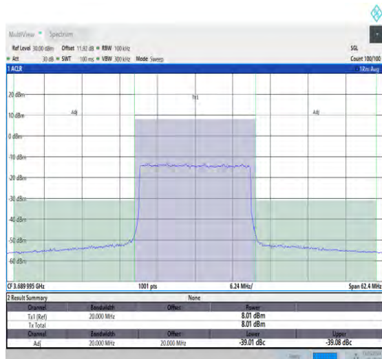
NTNV_N48_30_20_H_TID16_#1_-20_20
