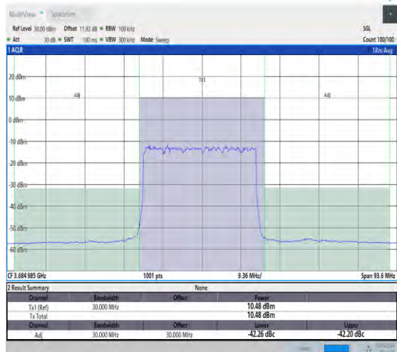
NTNV_N48_30_30_H_TID1_#1_-30_30
