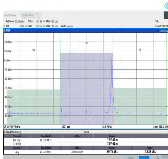
NTNV_N48_30_40_H_TID18_#1_-40_40
