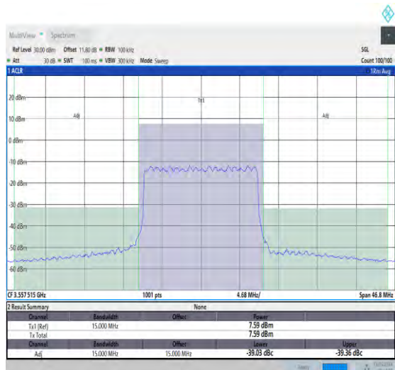
NTNV_N48_30_15_L_TID16_#1_-15_15
