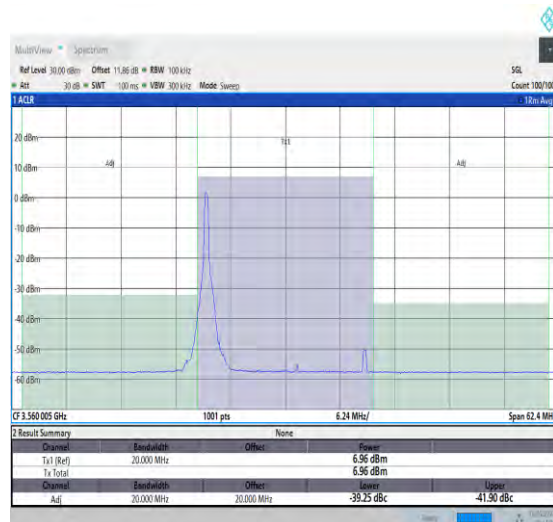
NTNV_N48_30_20_L_TID17_#1_-20_20
