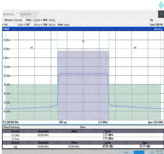
NTNV_N48_30_40_L_TID16_#1_-40_40
