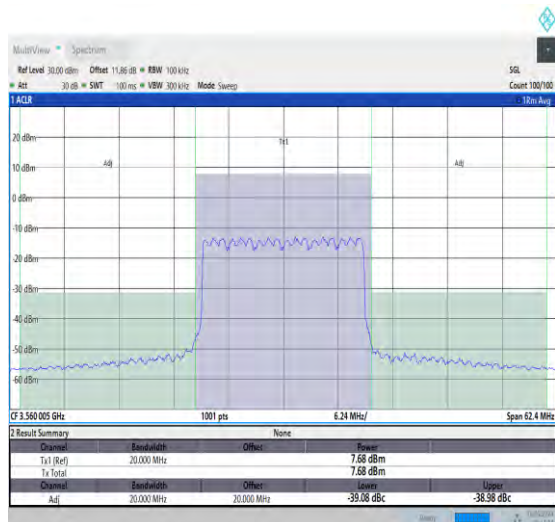
NTNV_N48_30_20_L_TID16_#1_-20_20
