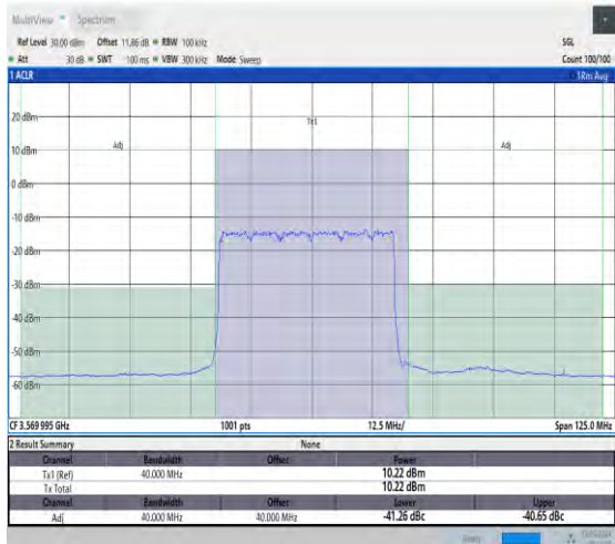
NTNV_N48_30_40_L_TID1_#1_-40_40
