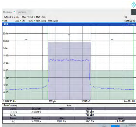
NTNV_N48_30_30_H_TID16_#1_-30_30
