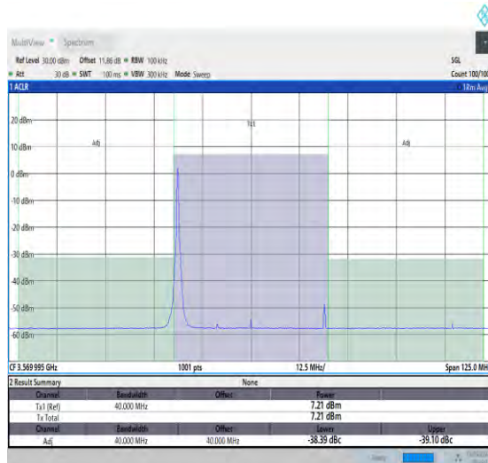
NTNV_N48_30_40_L_TID17_#1_-40_40
