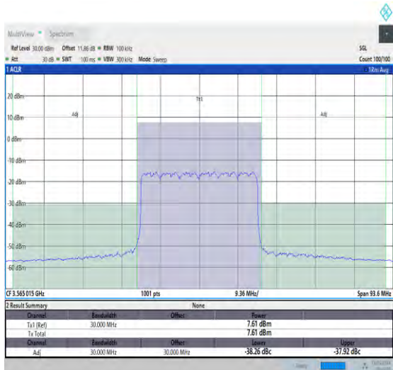
NTNV_N48_30_30_L_TID16_#1_-30_30
