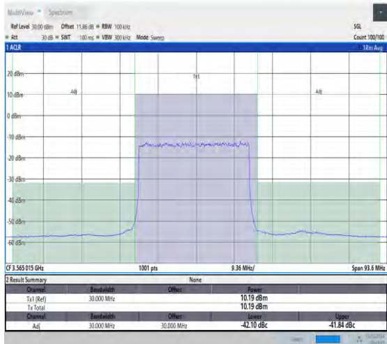
NTNV_N48_30_30_L_TID1_#1_-30_30
