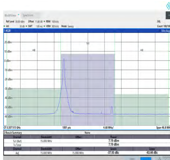
NTNV_N48_30_15_L_TID17_#1_-15_15
