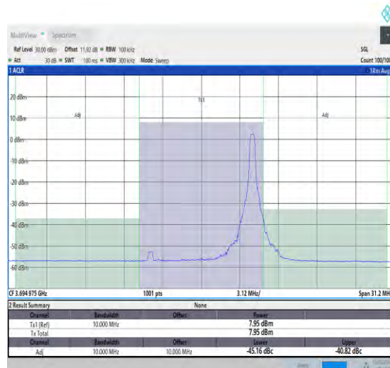
NTNV_N48_30_10_H_TID18_#1_-10_10
