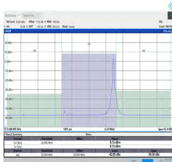
NTNV_N48_30_20_H_TID18_#1_-20_20
