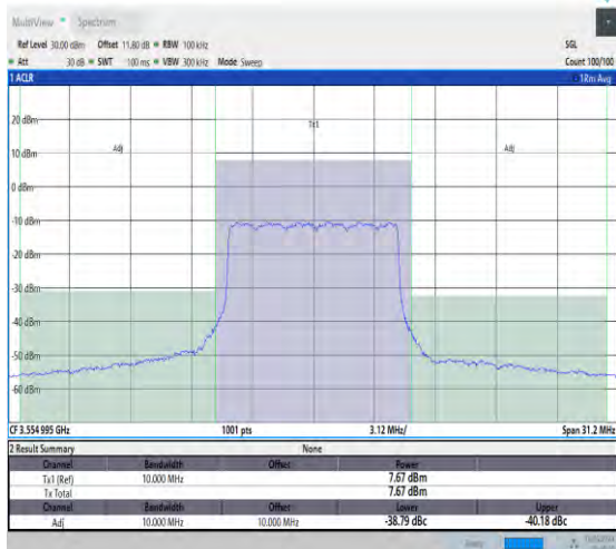
NTVN_N48_30_10_L_TID16_#1_-10_10
