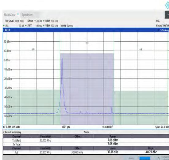
NTNV_N48_30_30_L_TID17_#1_-30_30
