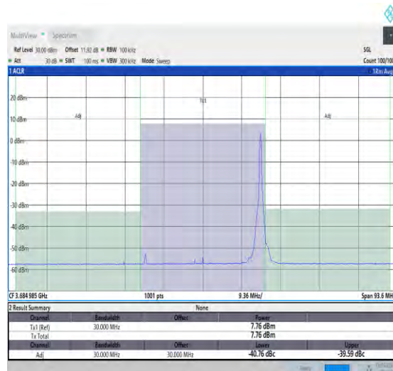
NTNV_N48_30_30_H_TID18_#1_-30_30
