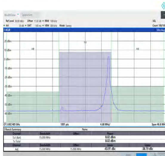
NTNV_N48_30_15_H_TID18_#1_-15_15
