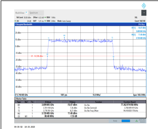
1-N78-3700-3800-30-80-L-7-CP-16QAM-Outer_Full-217@0-Ant0-77.363-80.480-≤80-PASS
