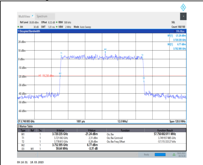
1-N78-3700-3800-30-60-M-9-CP-256QAM-Outer_Fu II-162@0-Ant0-57.75-59.640-≤60-PASS
