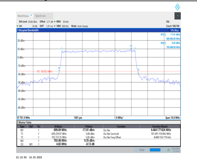
1-N12-PC3-15-5-L-6-CP-QPSK-Outer_Full-25@0-An t7-4.464-4.830-≤5-PASS
