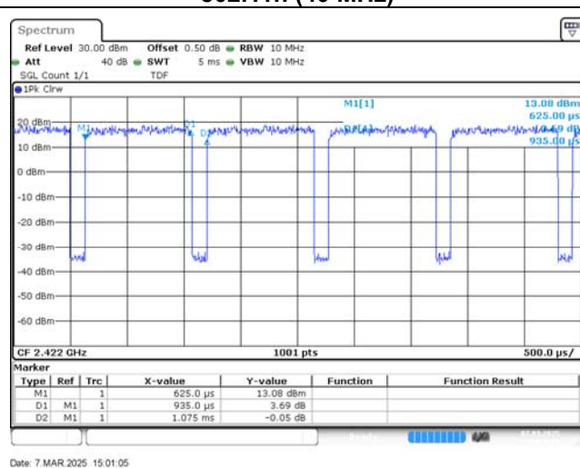
802.11n (40 MHz)
