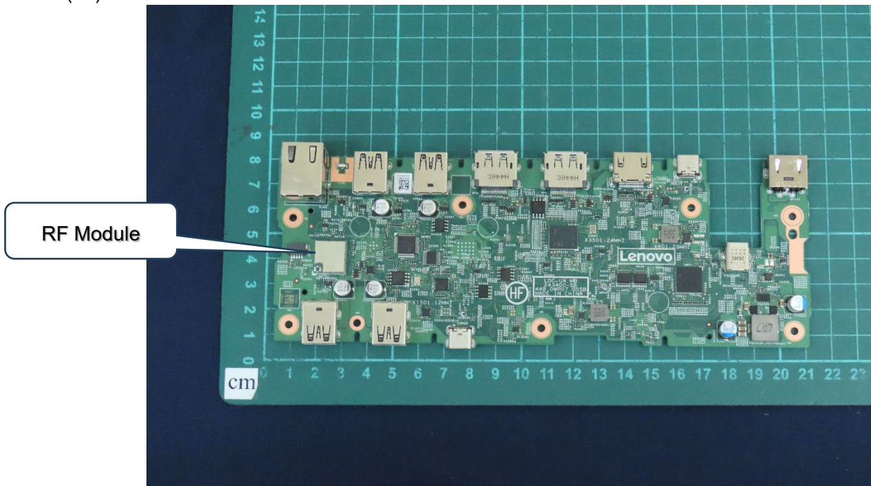
(17) EUT Photo
