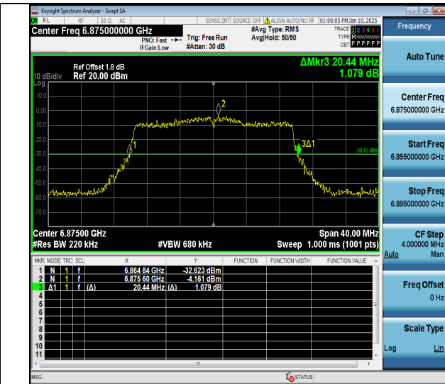
11ax20MIMO-Ant2-6875
