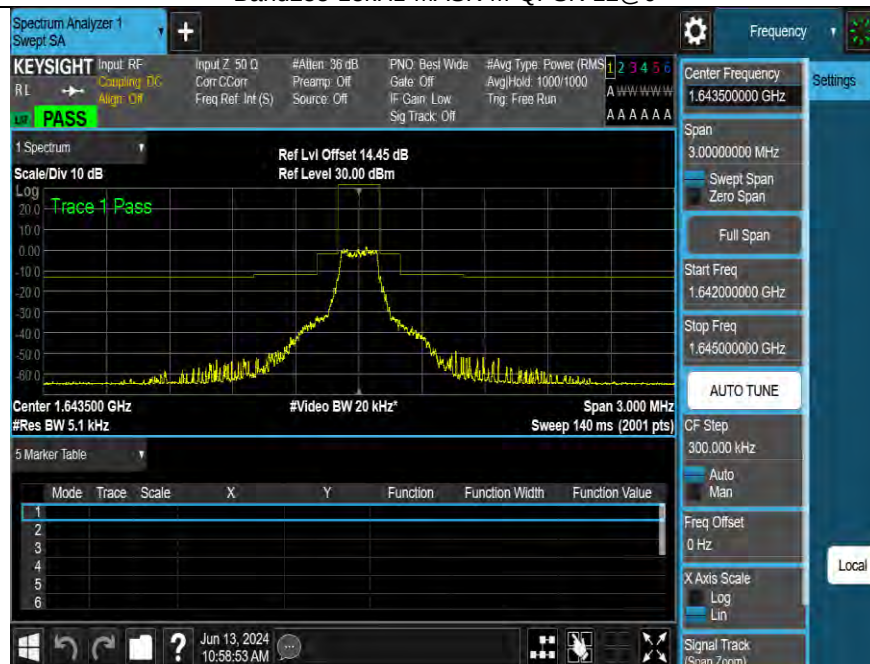
Band255-15kHz-MASK-M-QPSK-12@0
