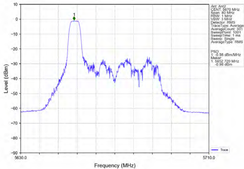
802.11ax(HE40) HCH 5670MHz RU52 Left MIMO NTN
