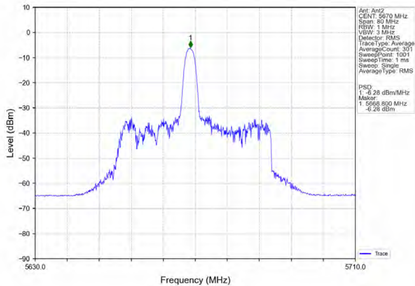
802.11ax(HE40) HCH 5670MHz RU26 Mid MIMO NTN
