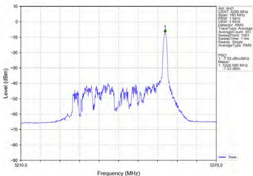
802.11ax(HE80) MCH 5290MHz RU26 Right Ant1 NTN
