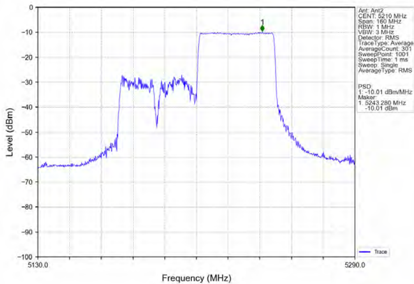
802.11ax(HE80) MCH 5210MHz RU484 Right MIMO NTVN
