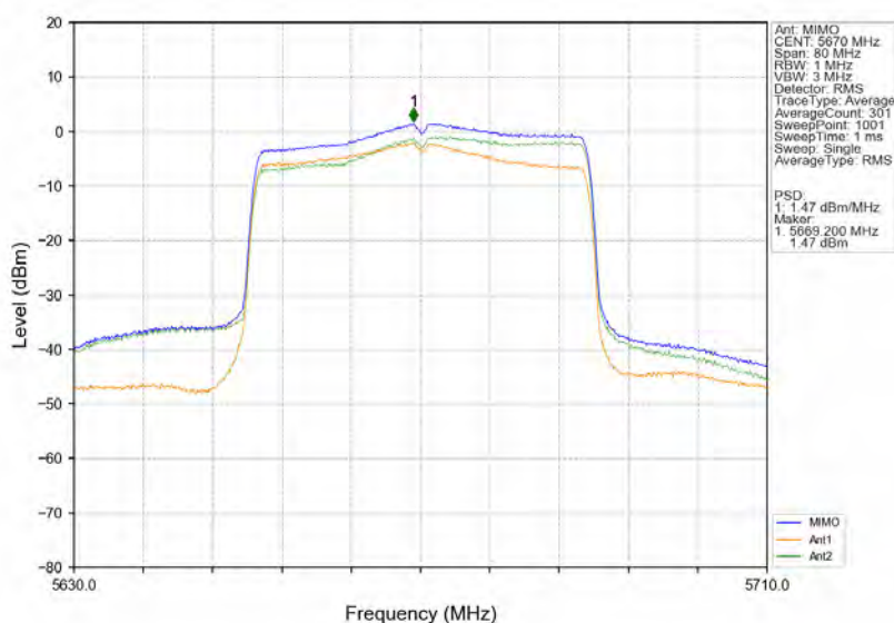
802.11ax(HE40) HCH 5670MHz RU484 Left MIMO NTN
