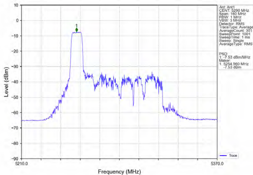
802.11ax(HE80) MCH 5290MHz RU106 Left Ant1 NTVN
