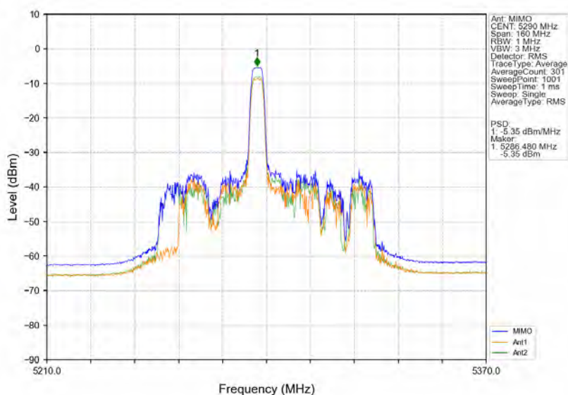
802.11ax(HE80) MCH 5290MHz RU52 Mid MIMO NTN
