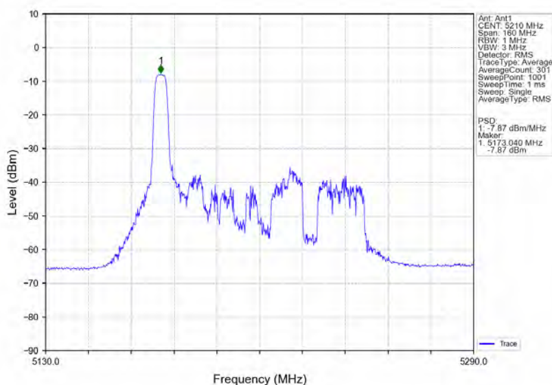
802.11ax(HE80) MCH 5210MHz RU52 Left Ant1 NTN
