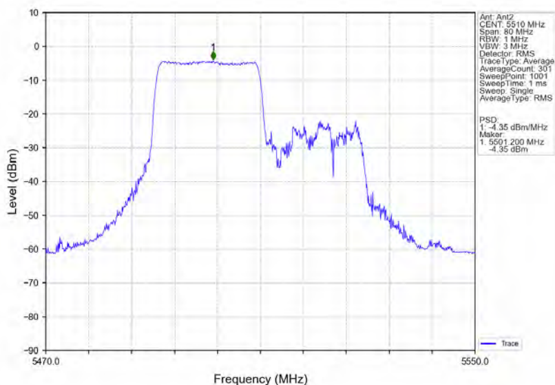
802.11ax(HE40) LCH 5510MHz RU242 Left MIMO NTN
