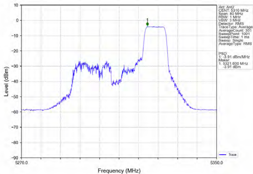
802.11ax(HE40) HCH 5310MHz RU106 Right Ant2 NTVN
