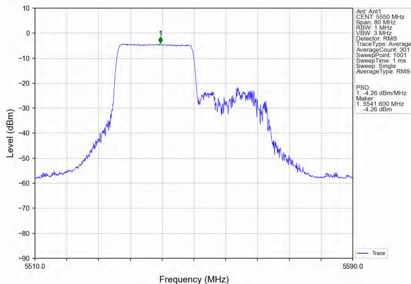
802.11ax(HE40) MCH 5550MHz RU242 Left Ant1 NTN
