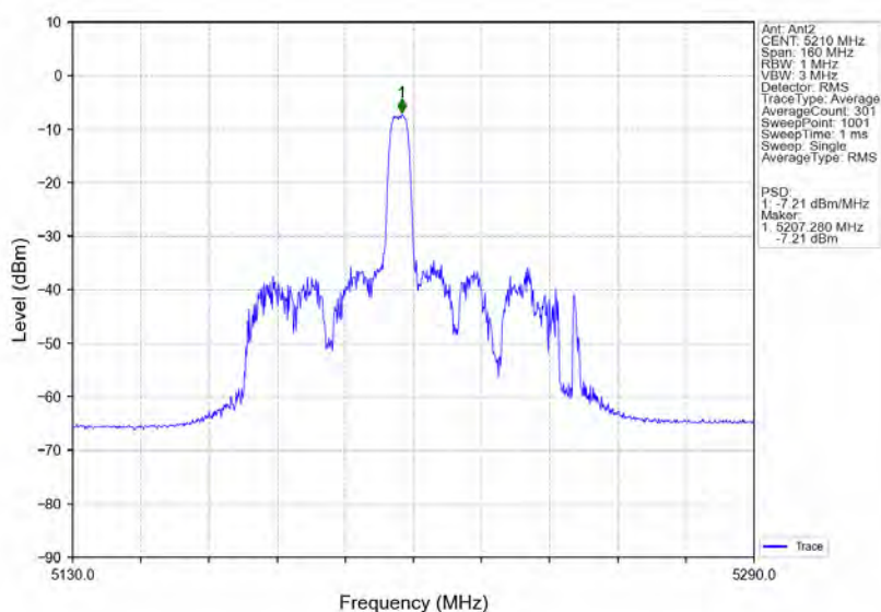
802.11ax(HE80) MCH 5210MHz RU52 Mid Ant2 NTN
