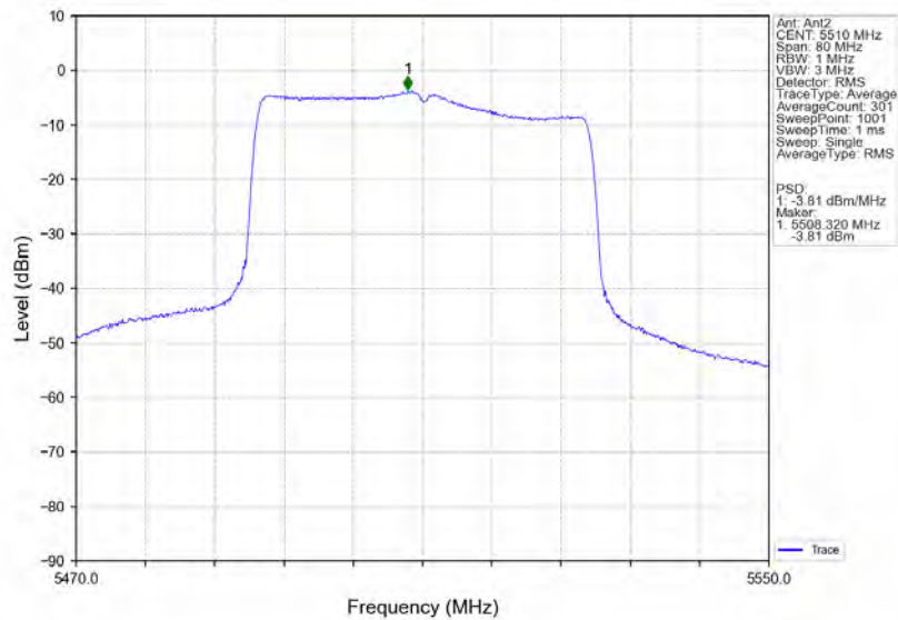
802.11ax(HE40) LCH 5510MHz RU484 Left MIMO NTN
