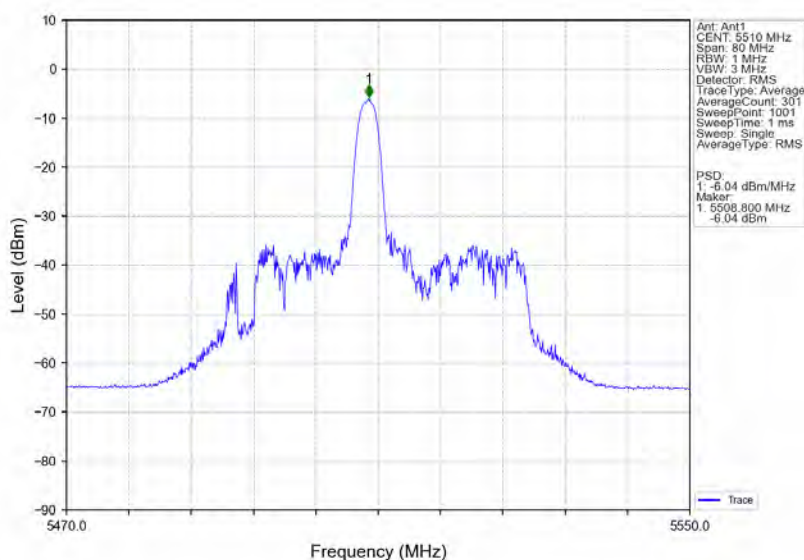
802.11ax(HE40) LCH 5510MHz RU26 Mid Ant1 NTN
