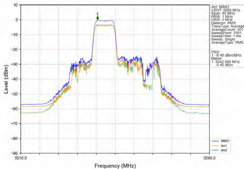
802.11ax(HE40) MCH 5550MHz RU106 Mid MIMO NTNv
