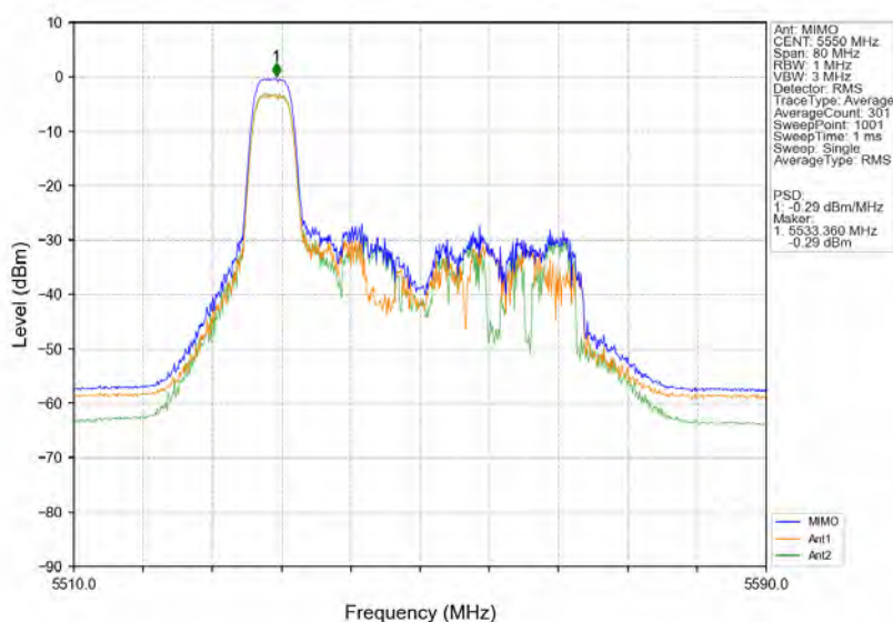
802.11ax(HE40) MCH 5550MHz RU52 Left MIMO NTN
