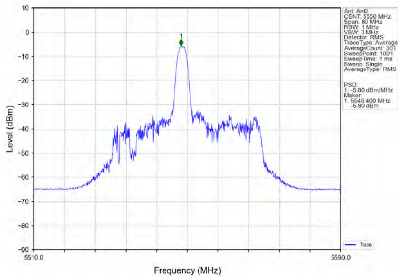
802.11ax(HE40) MCH 5550MHz RU26 Mid MIMO NTN
