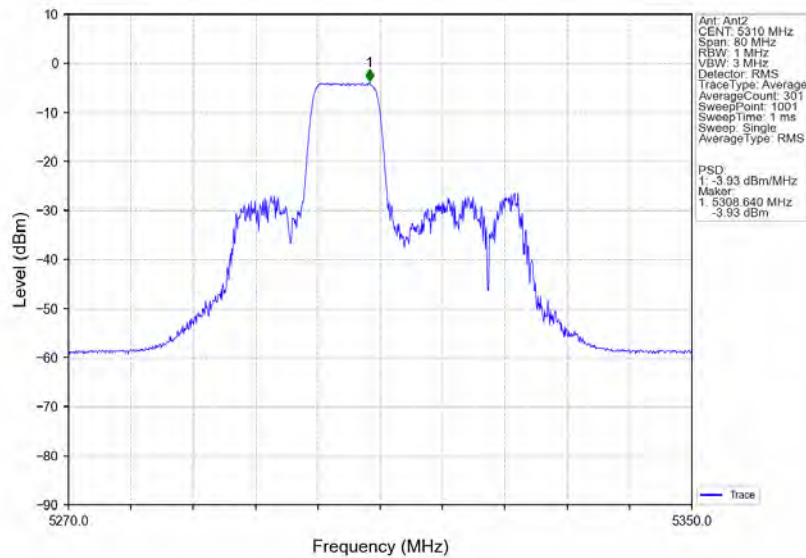
802.11ax(HE40) HCH 5310MHz RU106 Mid MIMO NTN
