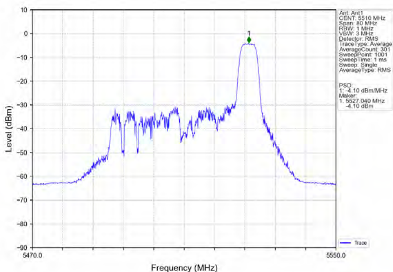
802.11ax(HE40) LCH 5510MHz RU52 Right Ant1 NTN
