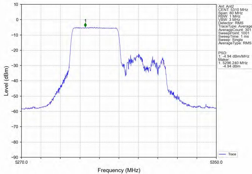
802.11ax(HE40) HCH 5310MHz RU242 Left MIMO NTN
