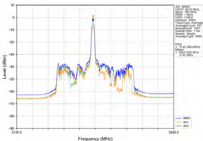
802.11ax(HE80) MCH 5210MHz RU26 Mid MIMO NTN
