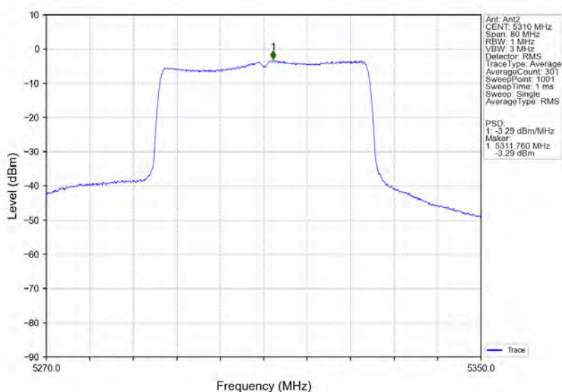
802.11ax(HE40) HCH 5310MHz RU484 Left MIMO NTN
