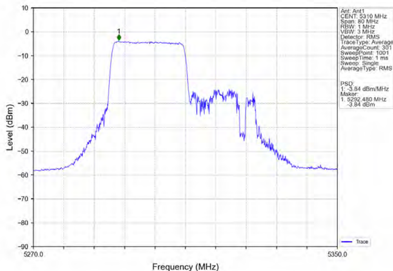
802.11ax(HE40) HCH 5310MHz RU242 Left Ant1 NTN
