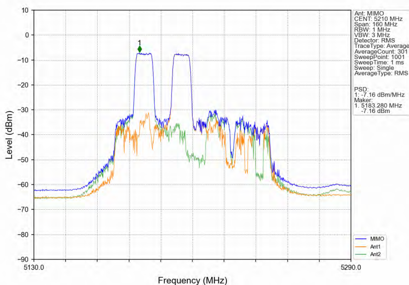
802.11ax(HE80) MCH 5210MHz RU106 Mid MIMO NTNv
