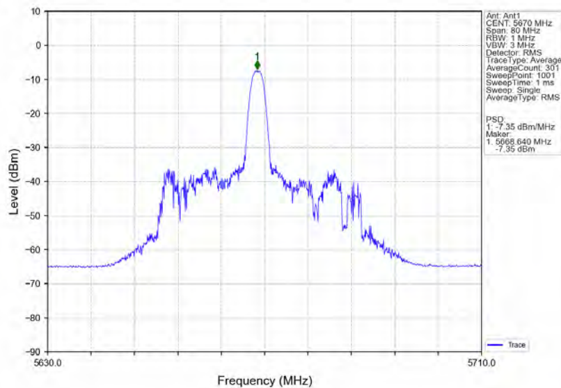
802.11ax(HE40) HCH 5670MHz RU26 Mid Ant1 NTNv
