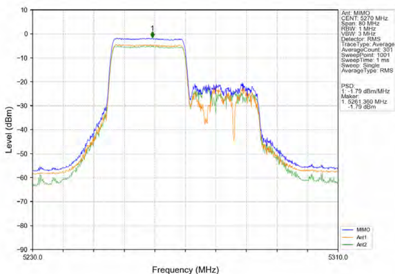
802.11ax(HE40) LCH 5270MHz RU242 Left MIMO NTN
