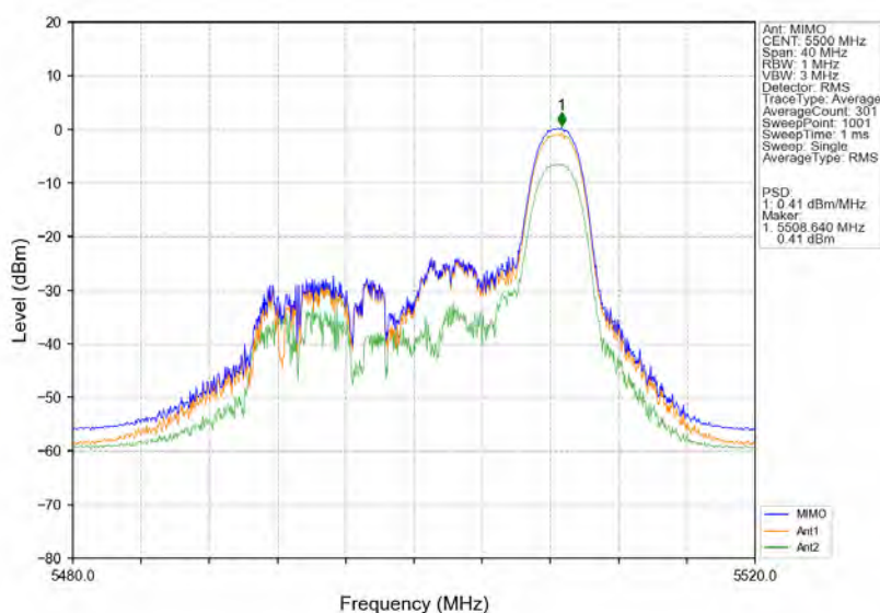
802.11ax(HE20) LCH 5500MHz RU26 Right MIMO NTNv
