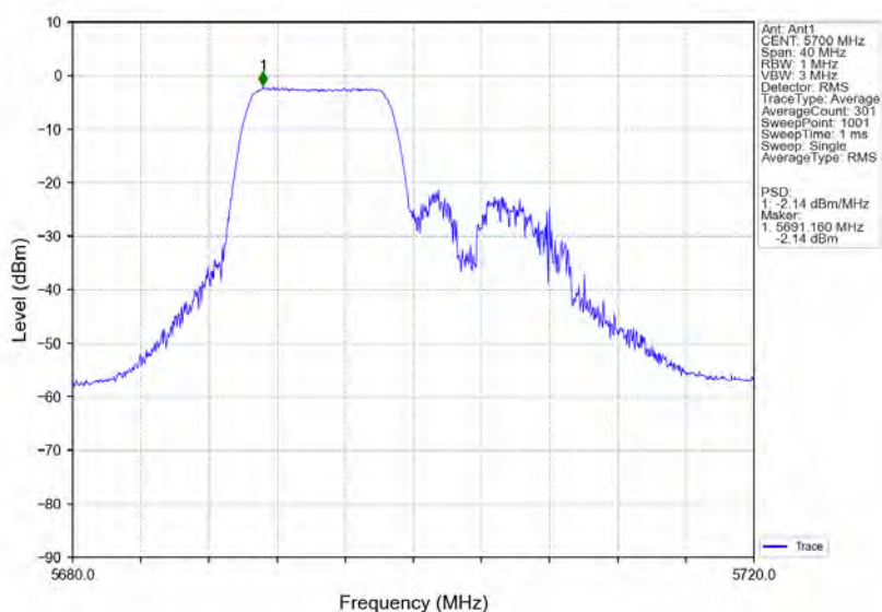
802.11ax(HE20) HCH 5700MHz RU106 Left Ant1 NTN
