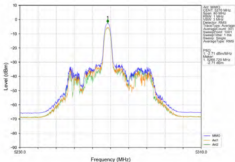
802.11ax(HE40) LCH 5270MHz RU26 Mid MIMO NTN
