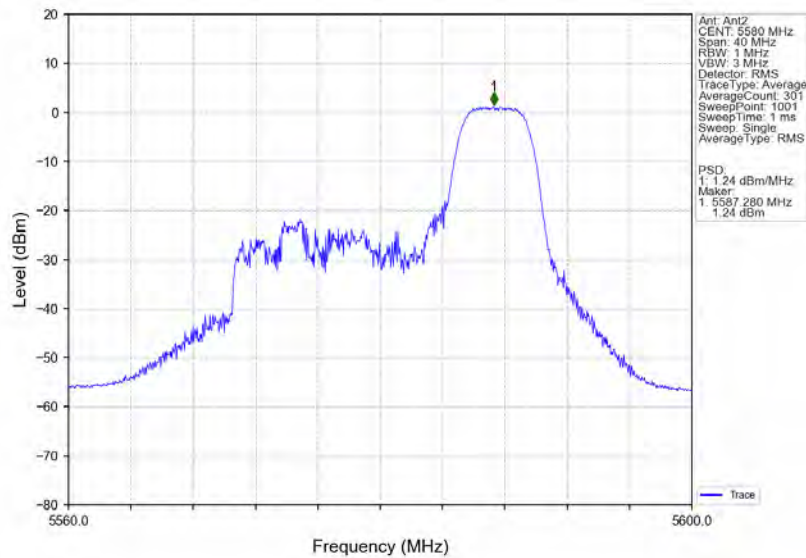
802.11ax(HE20) MCH 5580MHz RU52 Right MIMO NTN
