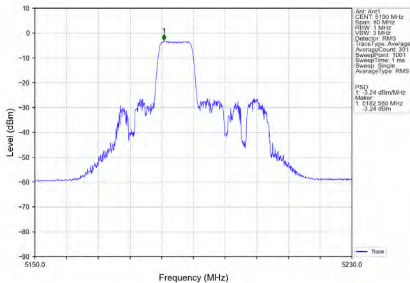
802.11ax(HE40) LCH 5190MHz RU106 Mid Ant1 NTN
