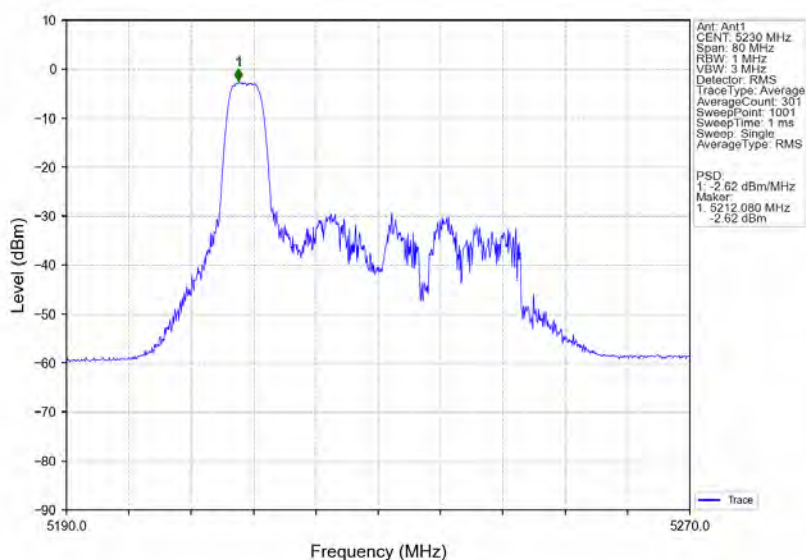
802.11ax(HE40) HCH 5230MHz RU52 Left Ant1 NTN
