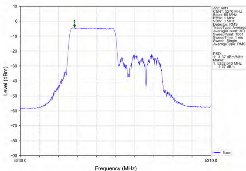
802.11ax(HE40) LCH 5270MHz RU242 Left Ant1 NTN
