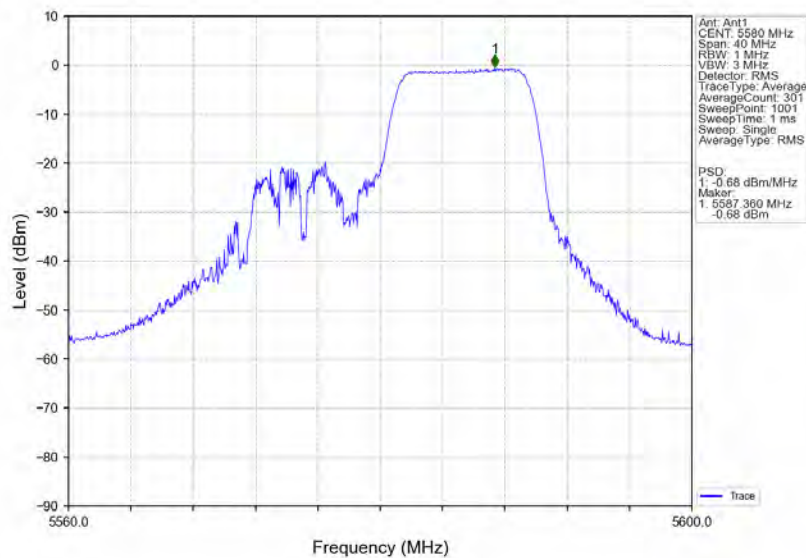
802.11ax(HE20) MCH_5580MHz RU106 Right Ant1 NTVN
