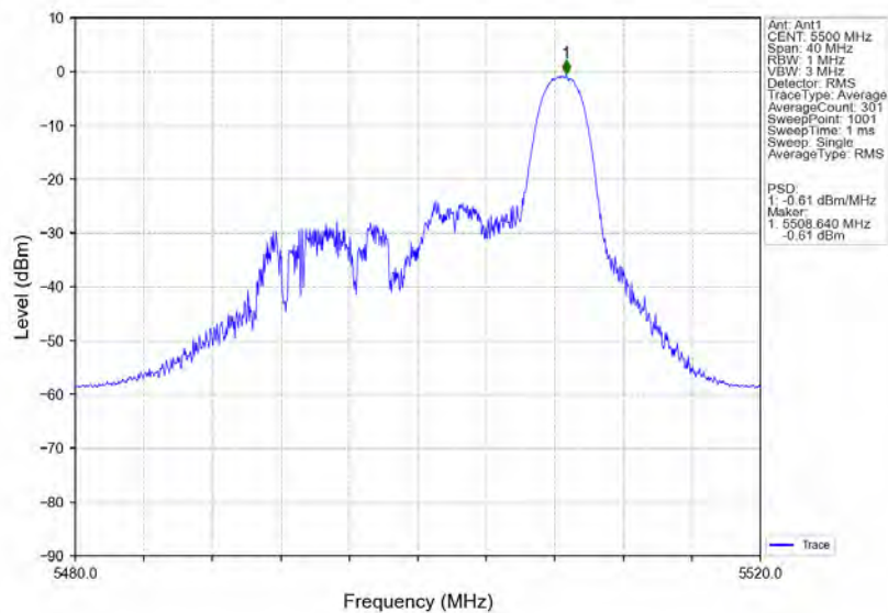
802.11ax(HE20) LCH 5500MHz RU26 Right Ant1 NTN
