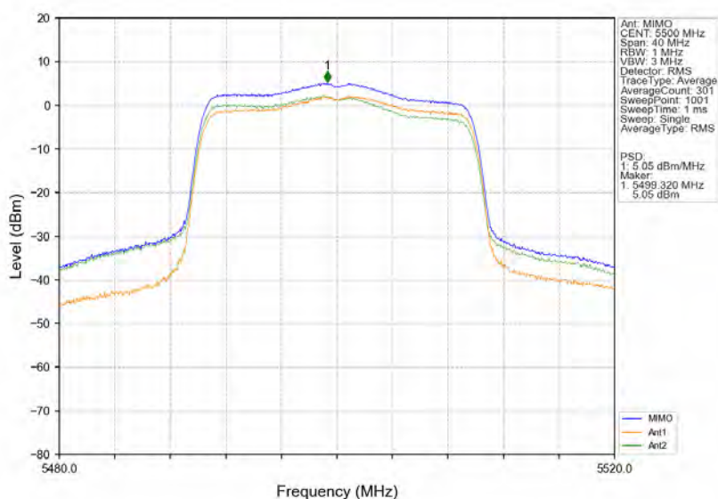
802.11ax(HE20) LCH 5500MHz RU242 Left MIMO NTN
