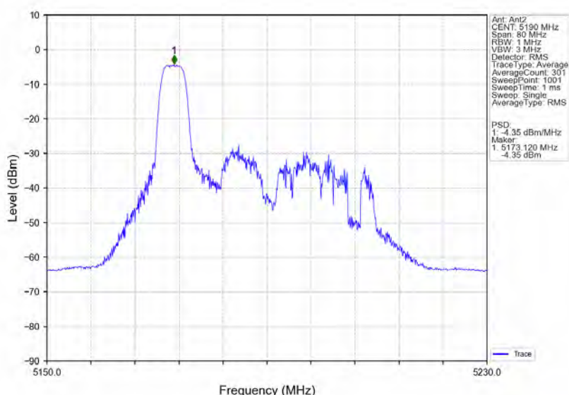
802.11ax(HE40) LCH 5190MHz RU52 Left MIMO NTNv
