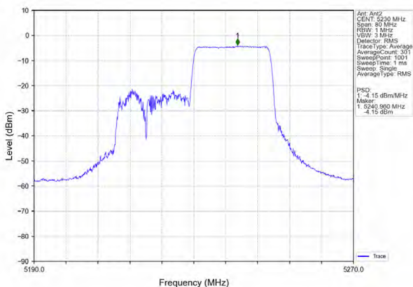
802.11ax(HE40) HCH 5230MHz RU242 Right Ant2 NTVN
