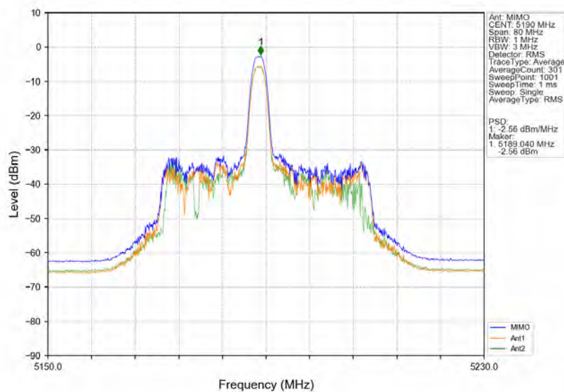
802.11ax(HE40) LCH 5190MHz RU26 Mid MIMO NTN
