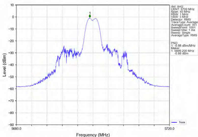
802.11ax(HE20) HCH 5700MHz RU26 Mid Ant2 NTN
