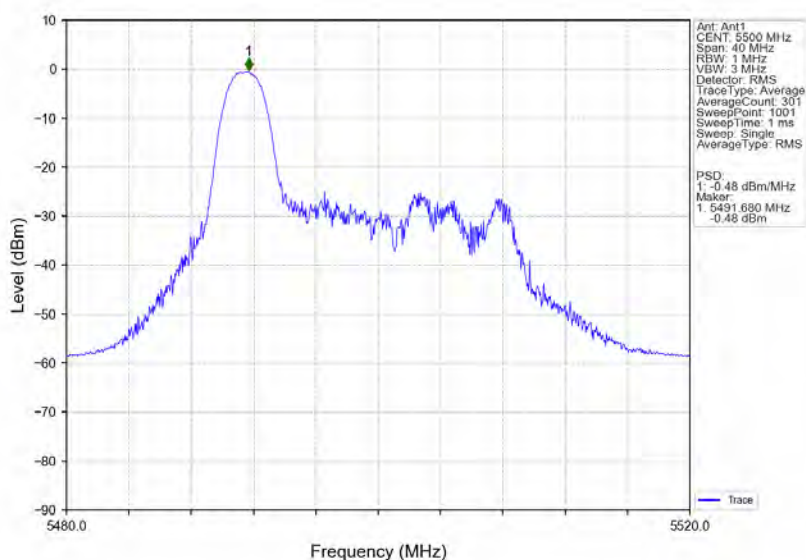
802.11ax(HE20) LCH 5500MHz RU26 Left Ant1 NTN
