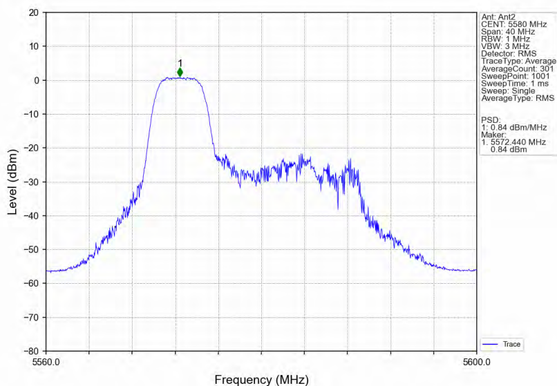
802.11ax(HE20) MCH 5580MHz RU52 Left MIMO NTN
