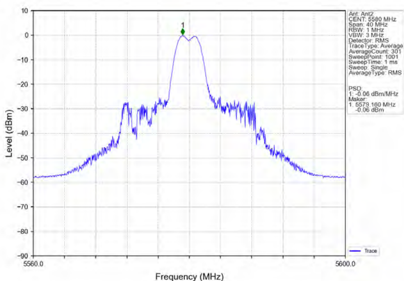
802.11ax(HE20) MCH 5580MHz RU26 Mid MIMO NTN
