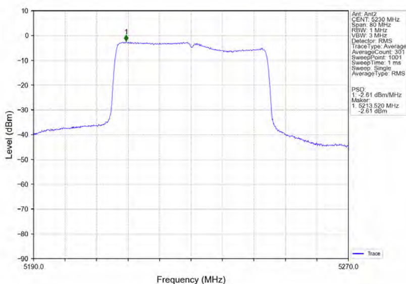
802.11ax(HE40) HCH 5230MHz RU484 Left MIMO NTN
