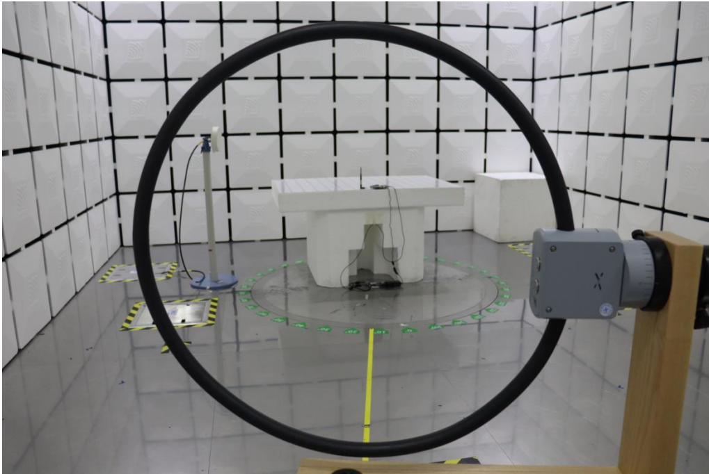
Wi-Fi_9KHz to 30MHz
