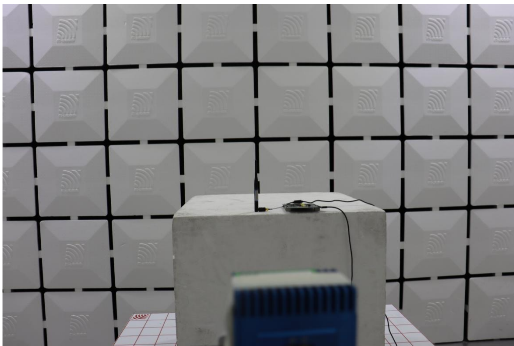
Wi-Fi_Above 18GHz
