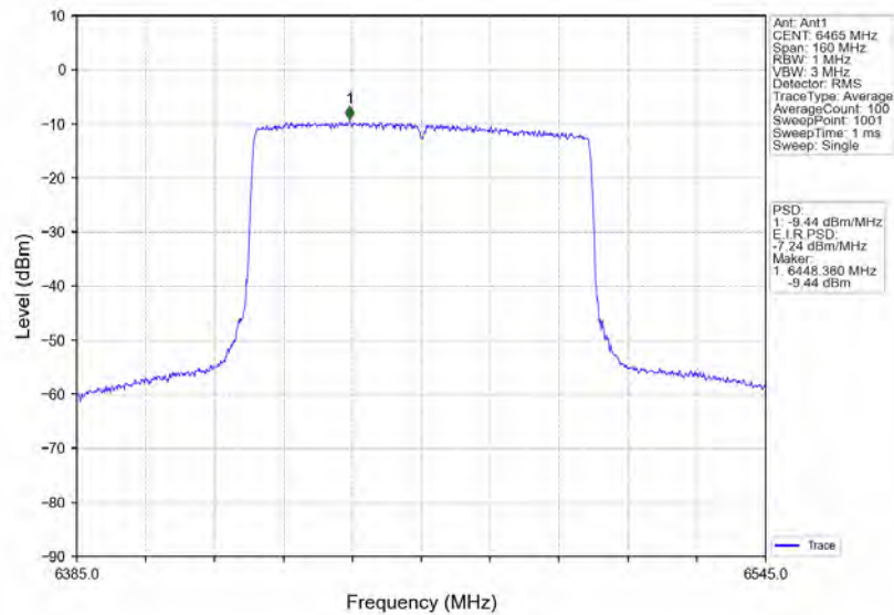
802.11ax(HEW80)_LCH_6465MHz_RU996_Left_Ant1_NTNV
