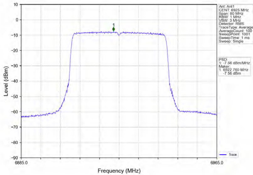
802.11ax(HEW40)_LCH_6925MHz_RU484_Left_Ant1_NTNV
