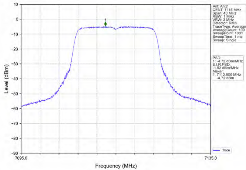
802.11a_HCH_7115MHz_Ant2_NTNV
