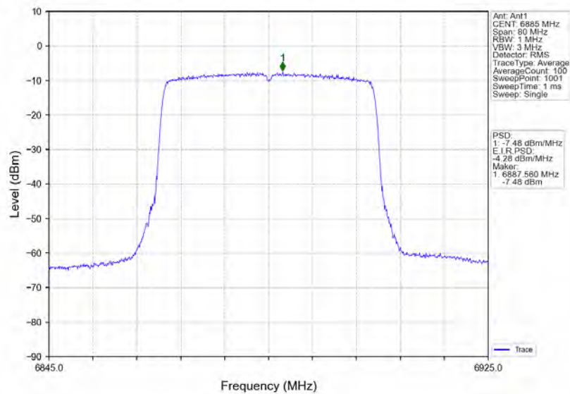
802.11ax(HEW40)_HCH_6885MHz_RU484_Left_Ant1_NTNV
