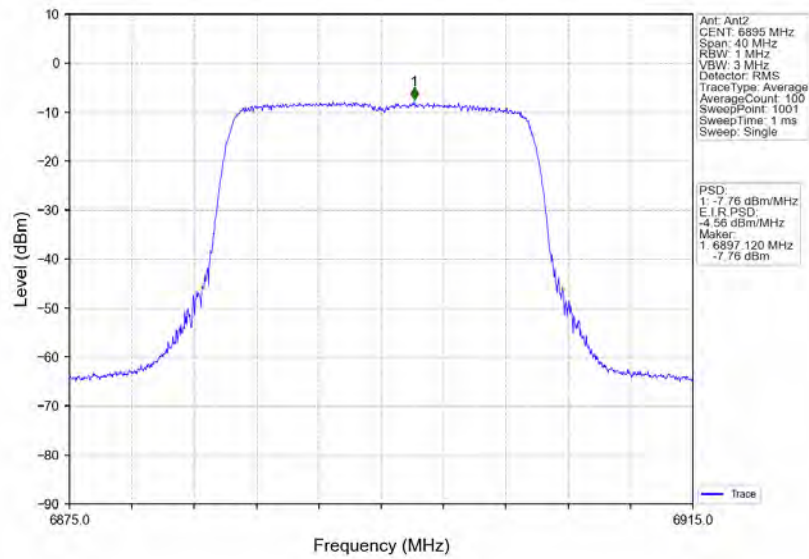
802.11ax(HEW20)_LCH_6895MHz_RU242_Left_Ant2_NTNV
