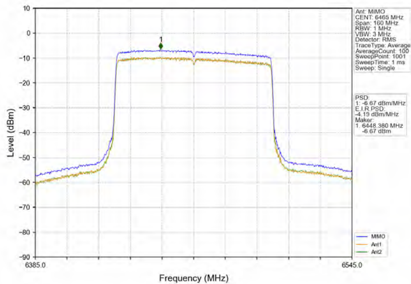
802.11ax(HEW80)_LCH_6465MHz_RU996_Left_MIMO_NTNV
