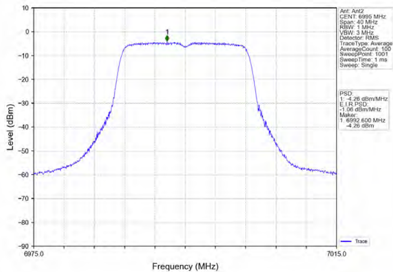
802.11a_MCH_6995MHz_Ant2_NTNV
