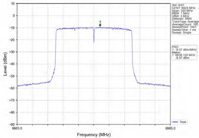
802.11ax(HEW160)_HCH_6825MHz_2xRU996_Left_Ant1_NTNV
