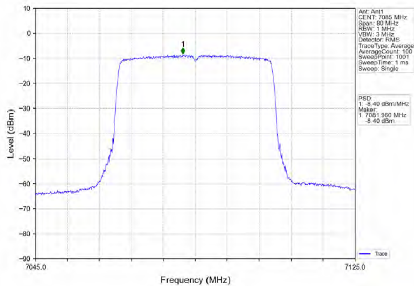
802.11ax(HEW40) HCH_7085MHz_RU484_Left_Ant1_NTNV
