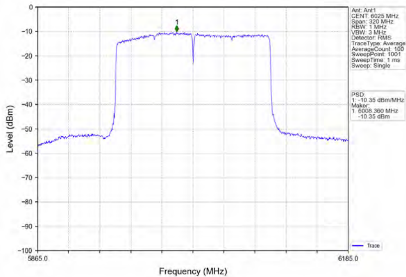
802.11ax(HEW160)_LCH_6025MHz_2xRU996_Left_Ant1_NTNV
