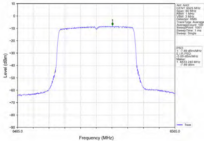
802.11ax(HEW40)_HCH_6525MHz_RU484_Left_Ant2_NTNV
