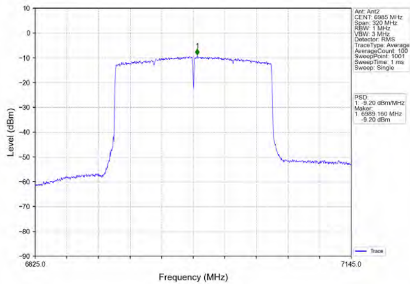
802.11ax(HEW160)_MCH_6985MHz_2xRU996_Left_Ant2_NTNV
