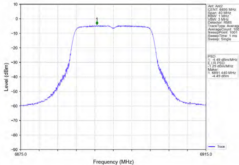
802.11a_LCH_6895MHz_Ant2_NTNV
