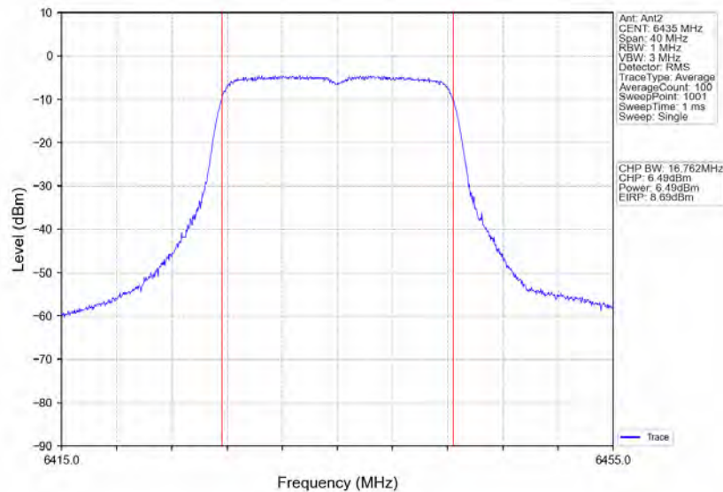
802.11a_LCH_6435MHz_Ant2_NTNV
