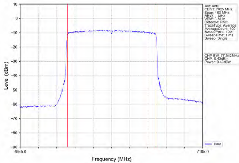
802.11ax(HEW80)_HCH_7025MHz_RU996_Left_Ant2_NTNV
