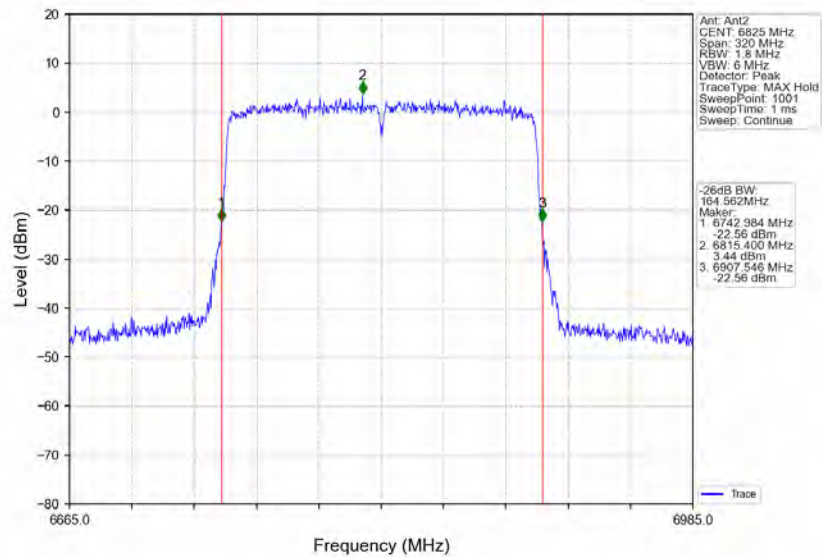
802.11ax(HEW160)_HCH_6825MHz_2xRU996_Left_Ant2_NTNV
