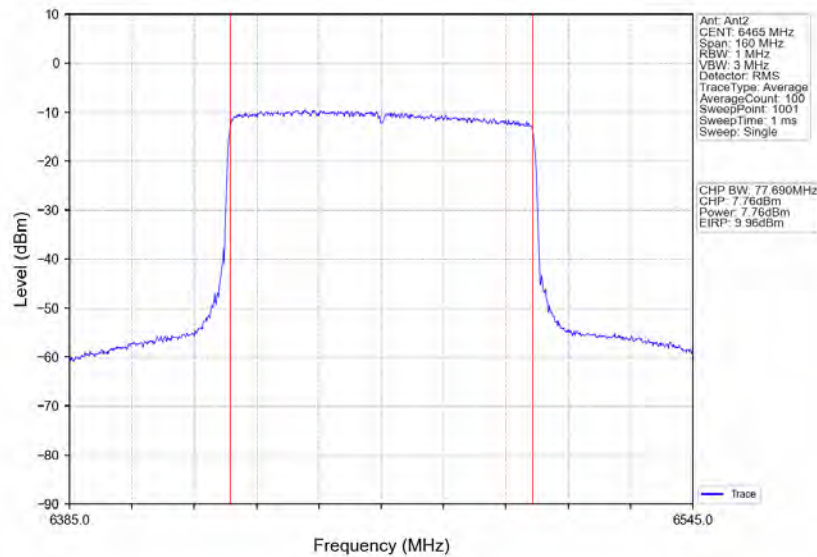
802.11ax(HEW80)_LCH_6465MHz_RU996_Left_Ant2_NTNV
