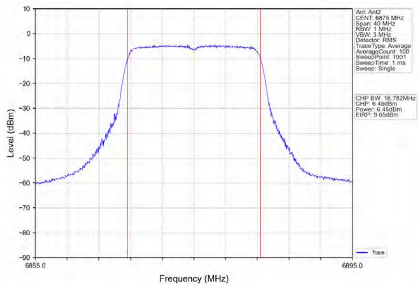
802.11a_HCH_6875MHz_Ant2_NTNV
