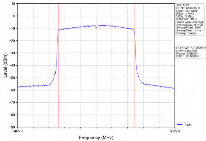
802.11ax(HEW80)_HCH_6545MHz_RU996_Left_Ant2_NTNV
