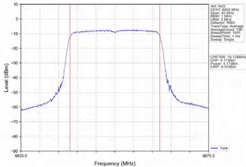
802.11ax(HEW20)_HCH_6855MHz_RU242_Left_Ant2_NTNV
