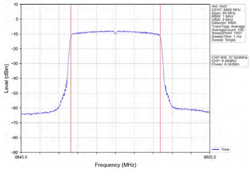
802.11ax(HEW40)_HCH_6885MHz_RU484_Left_Ant2_NTNV
