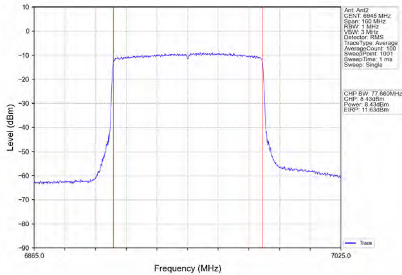
802.11ax(HEW80)_LCH_6945MHz_RU996_Left_Ant2_NTNV
