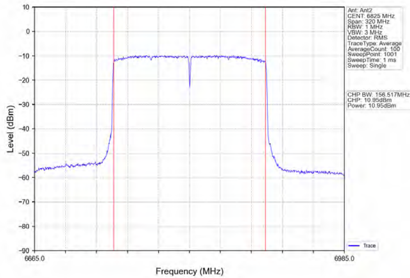
802.11ax(HEW160)_HCH_6825MHz_2xRU996_Left_Ant2_NTNV
