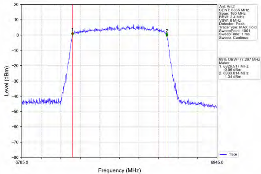
802.11ax(HEW80)_HCH_6865MHz_RU996_Left_Ant2_NTNV
