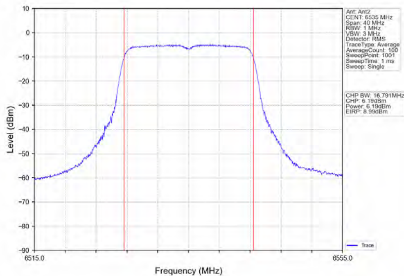
802.11a_LCH_6535MHz_Ant2_NTNV
