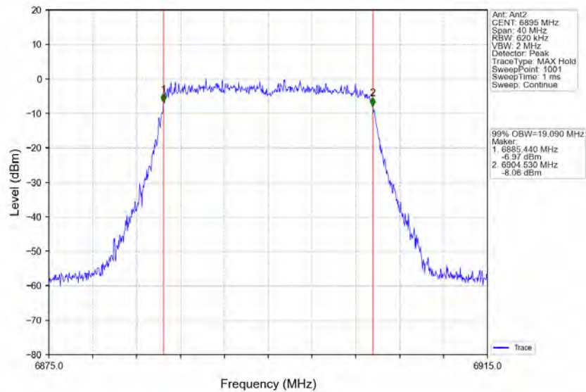
802.11ax(HEW20)_LCH_6895MHz_RU242_Left_Ant2_NTNV
