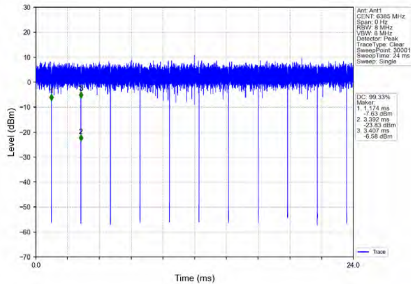
802.11ax(HEW80)_HCH_6385MHz_RU996_Left_Ant1_NTNV
