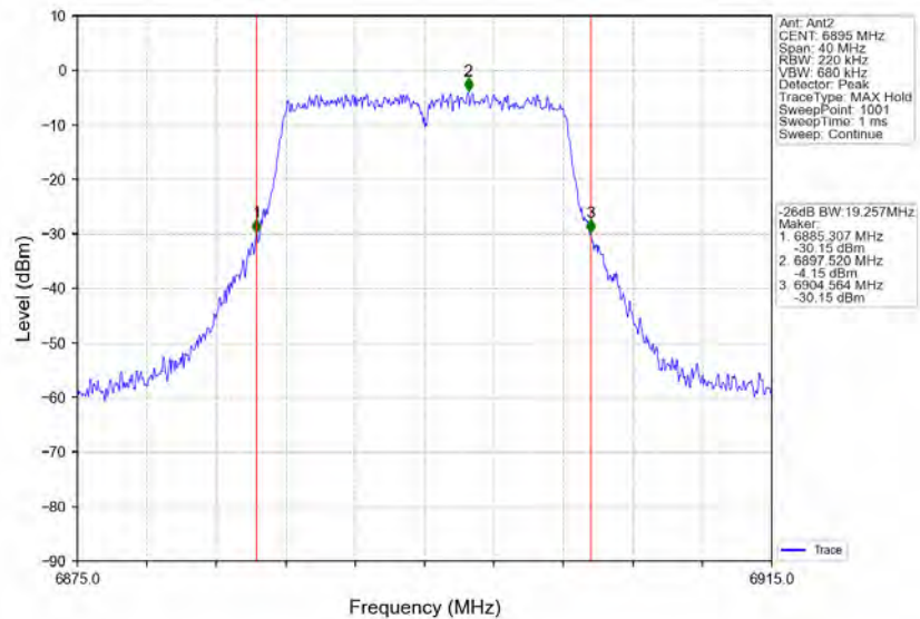
802.11a_LCH_6895MHz_Ant2_NTNV
