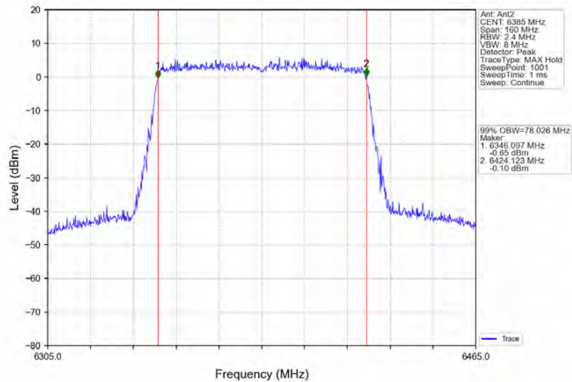
802.11ax(HEW80)_HCH_6385MHz_RU996_Left_Ant2_NTNV
