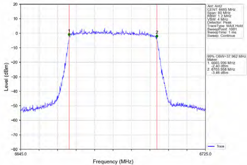
802.11ax(HEW40)_MCH_6685MHz_RU484_Left_Ant2_NTNV
