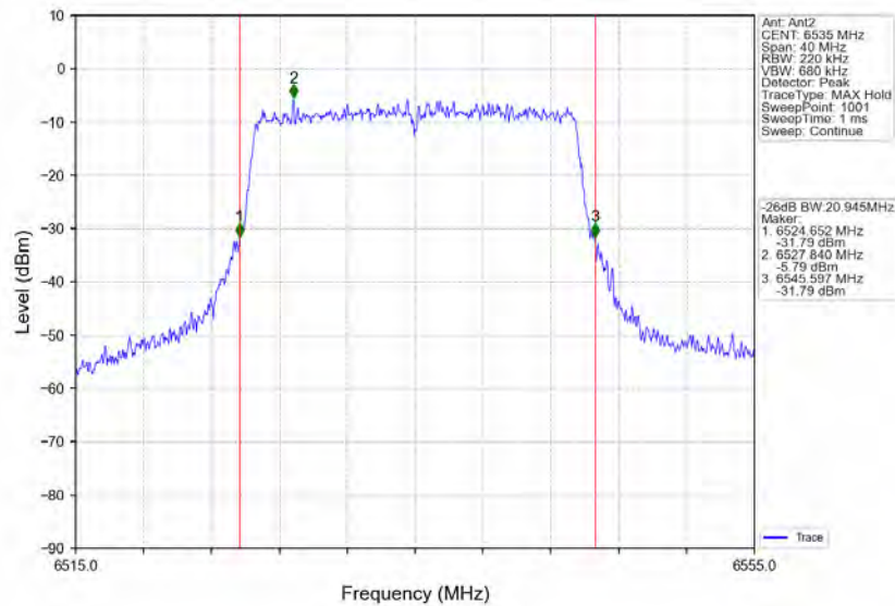
802.11ax(HEW20)_LCH_6535MHz_RU242_Left_Ant2_NTNV
