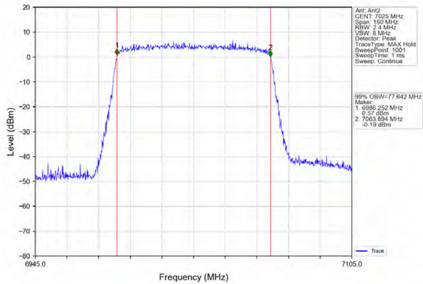
802.11ax(HEW80)_HCH_7025MHz_RU996_Left_Ant2_NTNV
