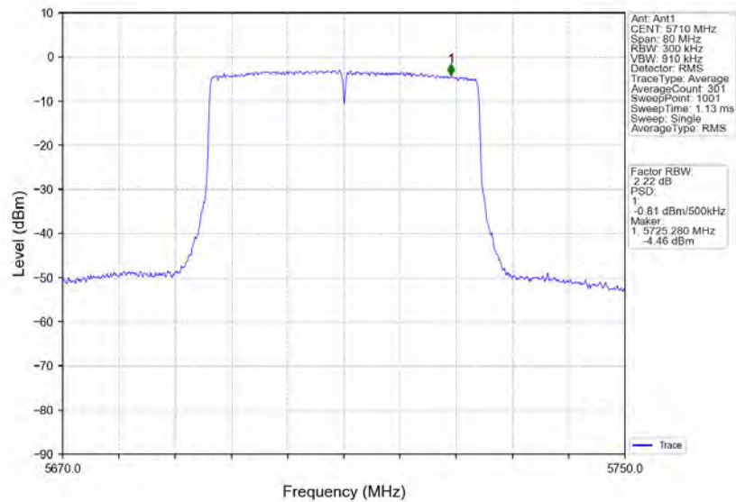
802.11ax(HEW40) HCH 5710MHz RU484 Left Ant1 NTN
