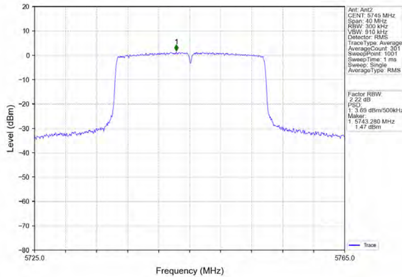
802.11ax(HEW20) LCH 5745MHz RU242 Left MIMO NTN
