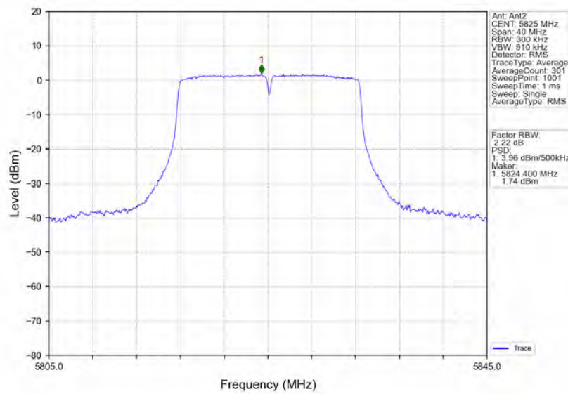
802.11a HCH 5825MHz Ant2 NTNv
