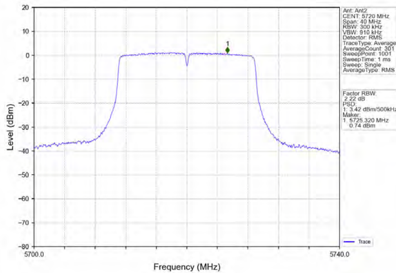
802.11n(HT20) HCH 5720MHz MIMO NTV
