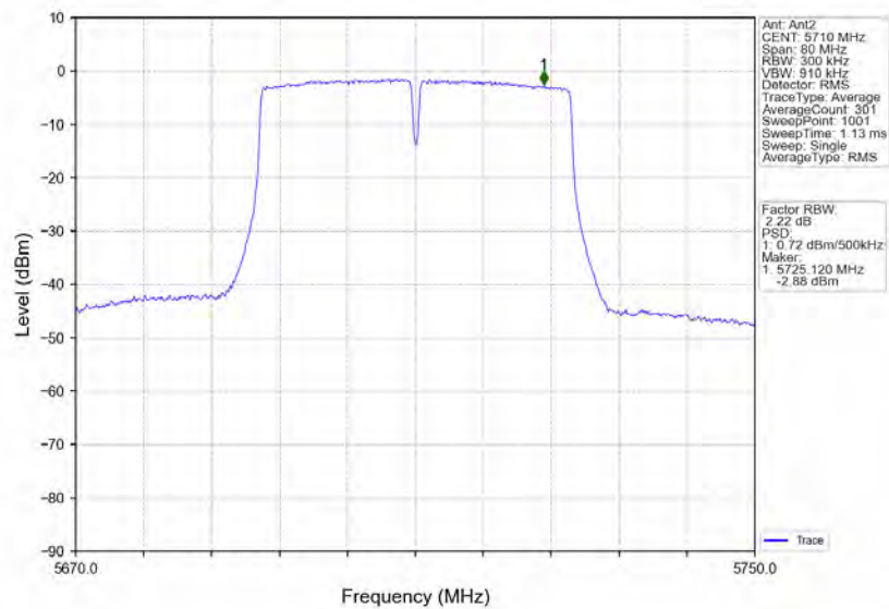
802.11n(HT40) HCH 5710MHz Ant2 NTN
