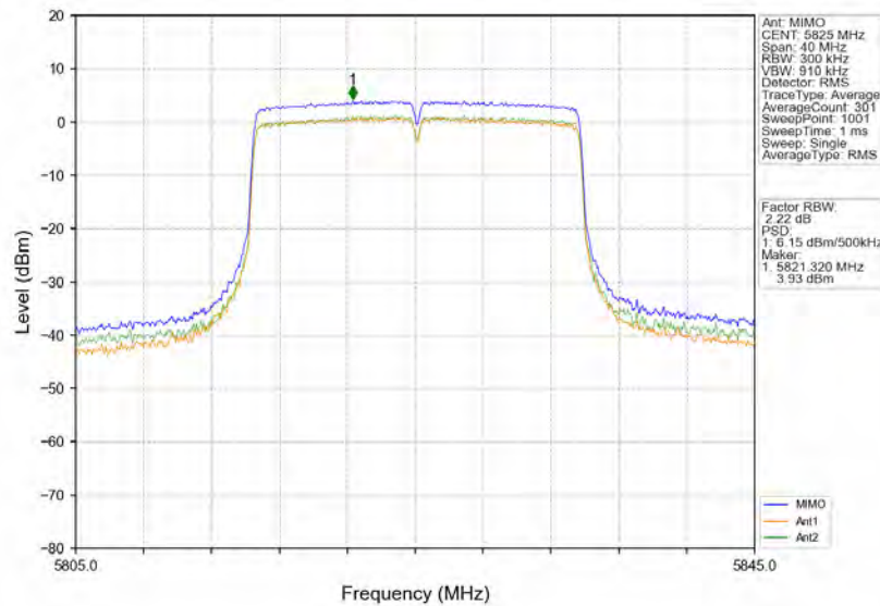
802.11ax(HEW20) HCH 5825MHz RU242 Left MIMO NTN
