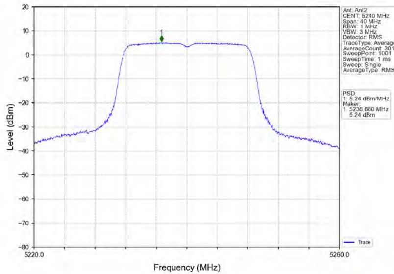
802.11a HCH 5240MHz Ant2 NTNv
