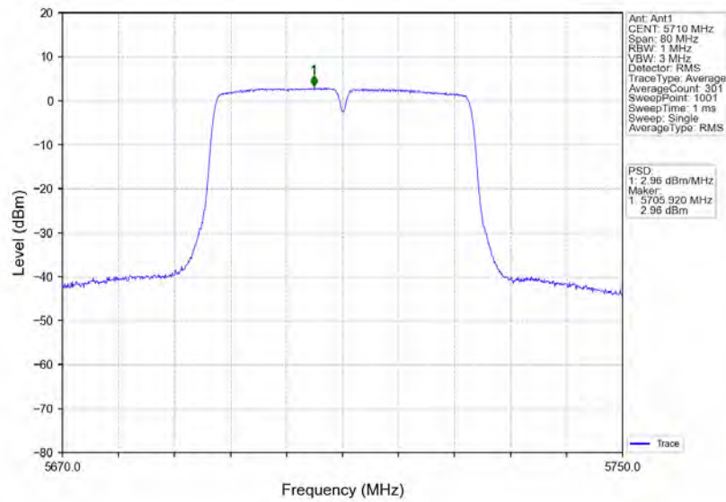
802.11n(HT40)_HCH_5710MHz_Ant1_NTNV
