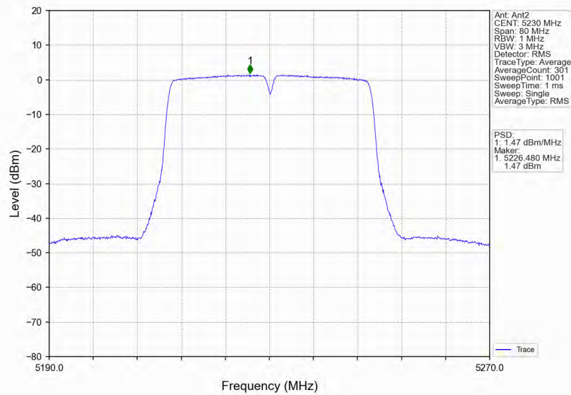
802.11n(HT40) HCH 5230MHz MIMO NTVN
