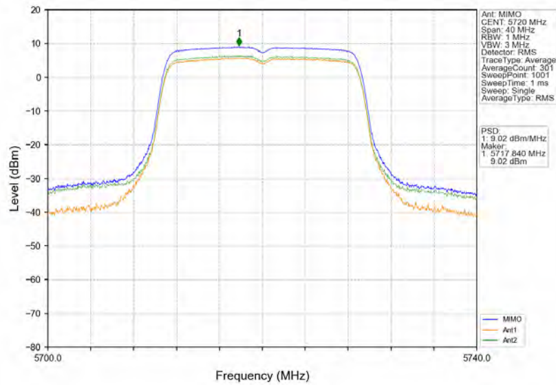
802.11n(HT20) HCH 5720MHz MIMO NTVN
