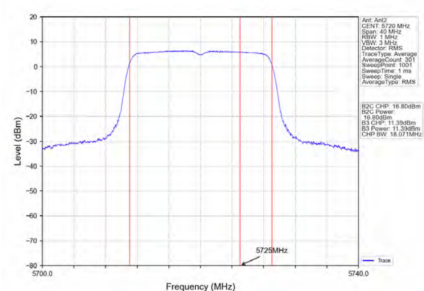
802.11n(HT20)_HCH_5720MHz_Ant2_NTN
