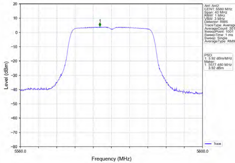
802.11n(HT20) MCH 5580MHz MIMO NTVN
