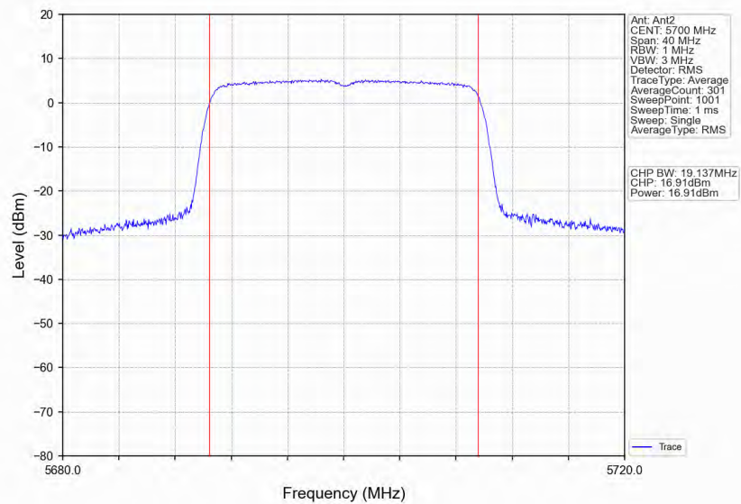
802.11ax(HEW20) HCH 5700MHz RU242 Left Ant2 NTNv
