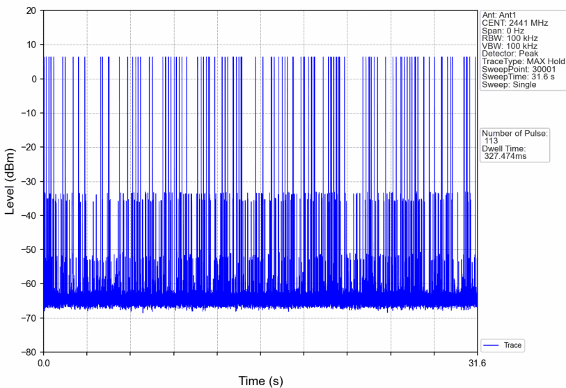
Pi/4DQPSK 2DH5 HOPP Ant1 NTNV
