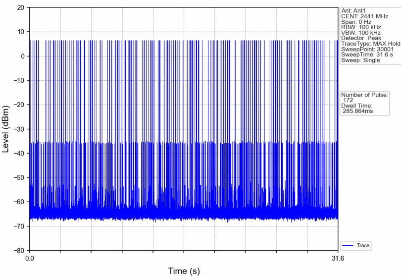
Pi/4DQPSK 2DH3 HOPP Ant1 NTNV
