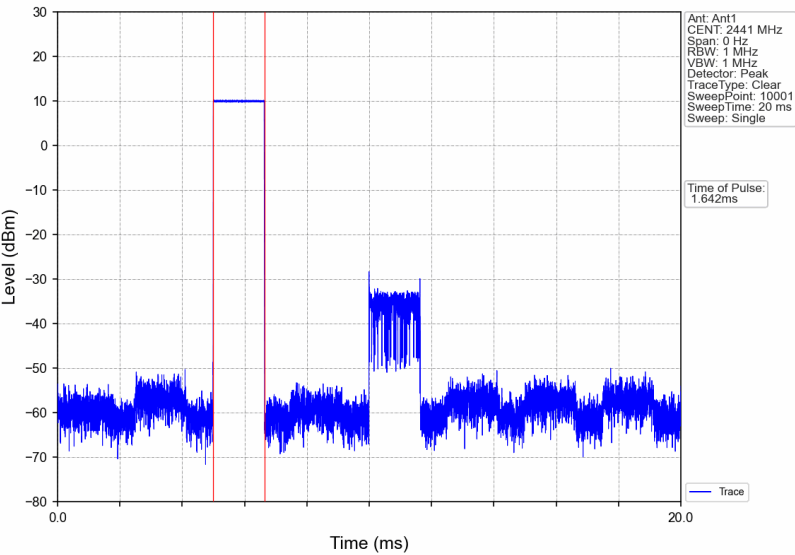
GFSK DH3 HOPP Ant1 NTNV
