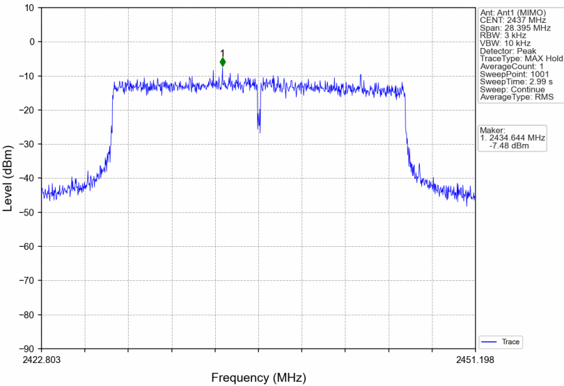
802.11ax(HEW20)_MCH_2437MHz_RU242_Left_Ant1 (MIMO)_NTNV
