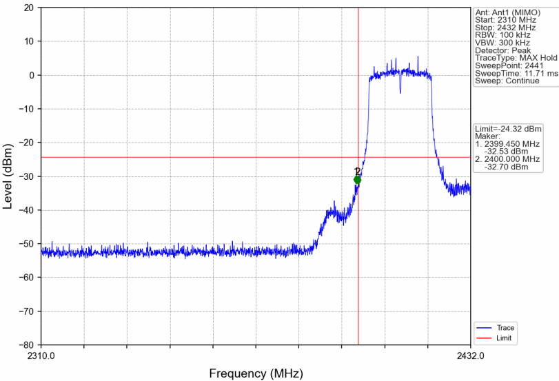
802.11n(HT20)_LCH_2412MHz_Ant1 (MIMO)_NTNV
