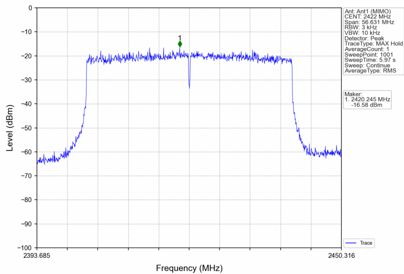
802.11ax(HEW40)_LCH_2422MHz_RU484_Left_Ant1 (MIMO)_NTNV
