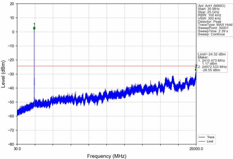
802.11n(HT20)_LCH_2412MHz_Ant1 (MIMO)_NTNV
