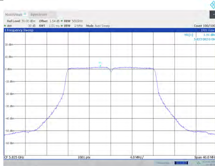
11a-CDD Ant0 5825
