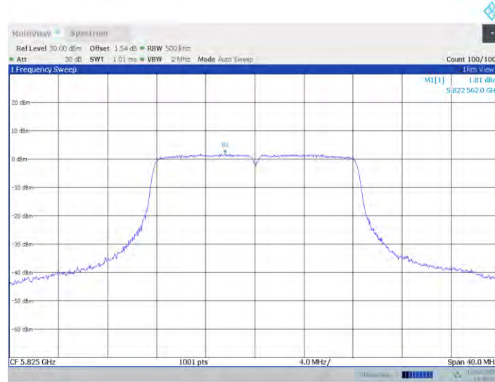
11a-CDD Ant1 5825
