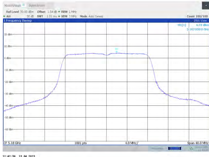
11a-CDD Ant1 5180
