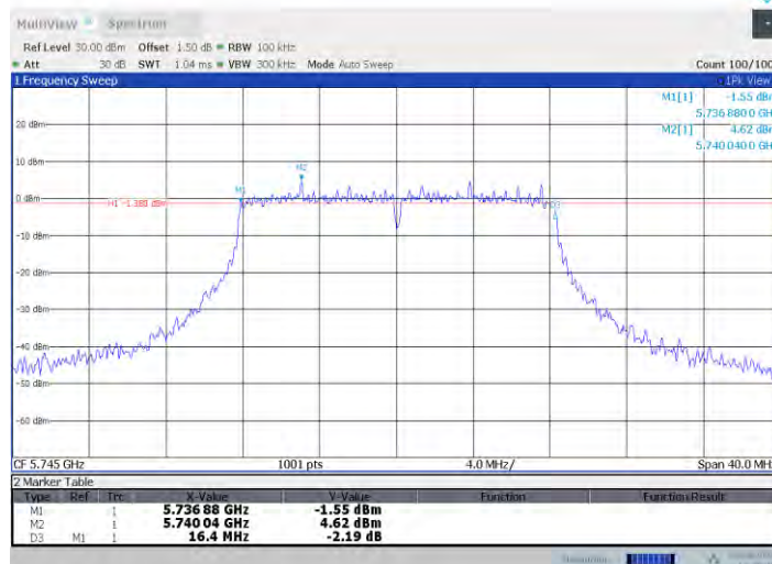
11a-CDD Ant1 5745
