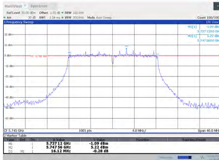
11a-CDD Ant1 5745
