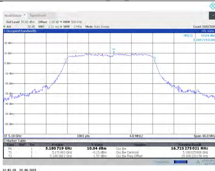
11a-CDD Ant1 5180
