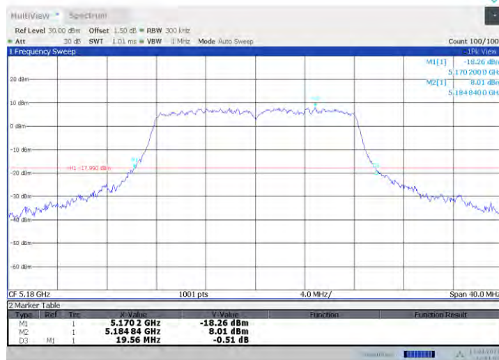
11a-CDD Ant1 5180
