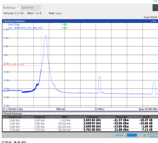
1-N78-3700-3800--30-30-L-4-CP-QPSK-Edge_1RB_L eft-1@0-Ant0-PASS-see graph
