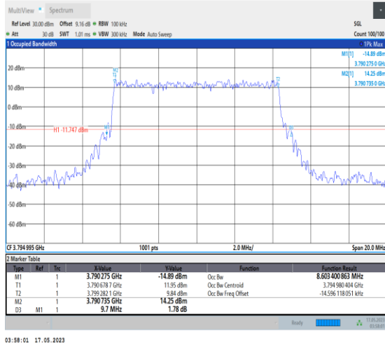
1-N78-3700-3800-PC1-30-10-H-3-DFT-16QAM-Outer_Full-24@0-Ant0-8.603-9.700-≤10-PASS
