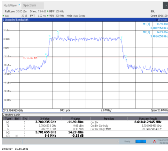
1-N78-3700-3800--30-10-L-1-DFT-QPSK-Out_ Full-24@0-Ant0-8.618-9.600≤10-PASS
