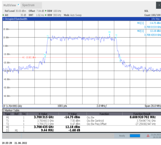
1-N78-3700-3800--30-10-L-3-DFT-16QAM-Out_ Full-24@0-Ant0-8.609-9.440≤10-PASS
