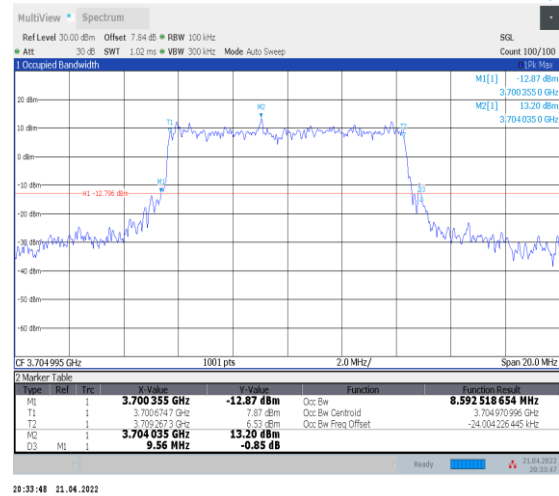
1-N78-3700-3800--30-10-L-4-DFT-64QAM-Out_ Full-24@0-Ant0-8.593-9.560≤10-PASS
