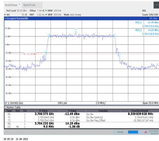
1-N78-3700-3800--30-10-L-2-DFT-PI2BPSK-Out_ Full-24@0-Ant0-8.56-9.500≤10-PASS
