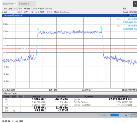
1-N78-3450-3550--30-50-H-8-CP-64QAM-Outer_Full -133@0-Ant0-47.222-49.200-≤50-PASS
