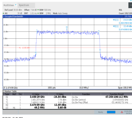
1-N78-3450-3550--30-50-L-7-CP-16QAM-Outer_Full -133@0-Ant0-47.354-49.300-≤50-PASS
