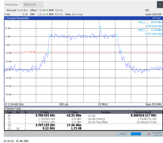
1-N77-3700-3980--30-10-L-2-DFT-PI2BPSK-Outter_Full -24@0-Ant0-8.569-9.220-≤10-PASS
