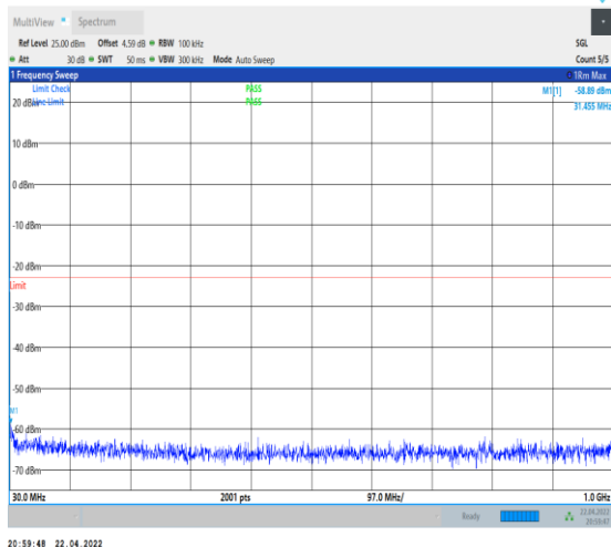
1-N66-PC3-15-40-M-1-DFT-PI2BPSK-Inner_1RB_L eft-1@1-30-1000-Ant0--58.89--23-PASS
