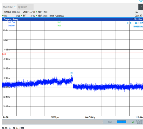
1-N66-PC3-15-40-M-1-DFT-PI2BPSK-Inner_1RB_L eft-1@1-3000-12000-Ant0--38.11--13-PASS
