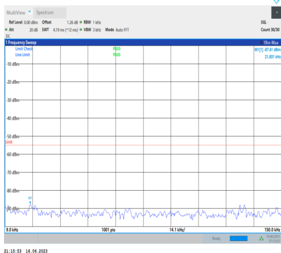
1-N41-PC1-30-100-L-1-DFT-QPSK-Edge_1RB_Left -1@0-0.009-0.15-Ant0-0.02--87.61--55-PASS
