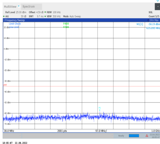
1-N38--30-40-L-1-DFT-PI2BPSK-Inner_1RB_Left-1 @1-30-1000-Ant0--58.19--35-PASS
