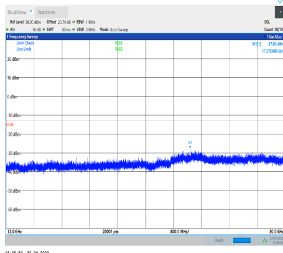
1-N25--15-40-L-1-DFT-PI2BPSK-Inner_1RB_Left-1@ 1-12000-20000-Ant0--27.80--13-PASS
