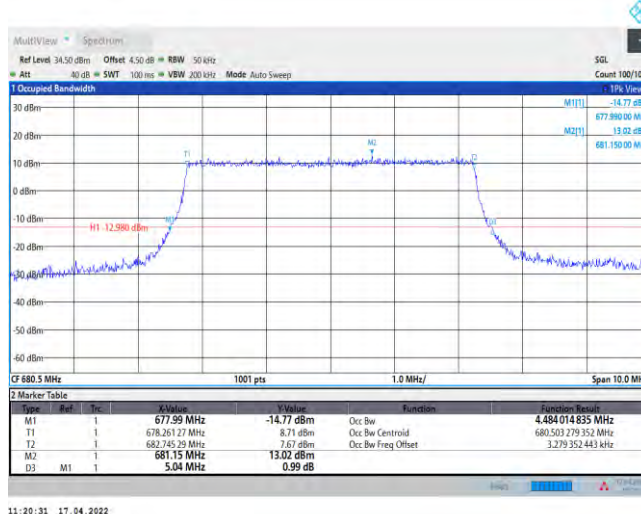
Band71-5MHz-QPSK-133297-25RB#0
