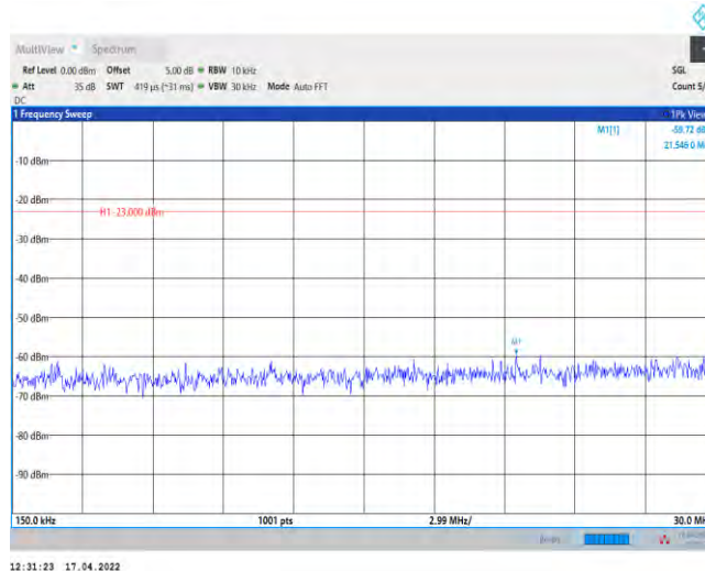
Band66-20MHz-QPSK-132072-1RB#0-Range2:0.15~30MHz
