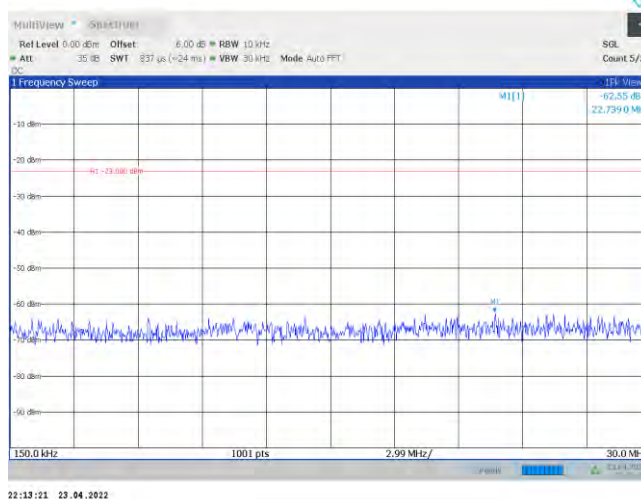
Band43-20MHz-QPSK-44690-1RB#0-Range2:0.15~30MHz
