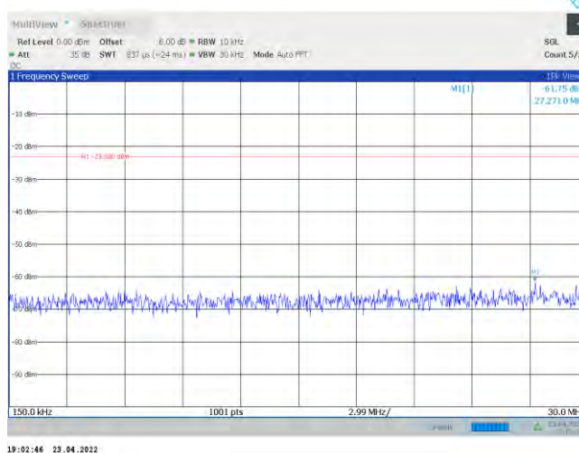
Band42-20MHz-QPSK-42190-1RB#0-Range2:0.15~30MHz
