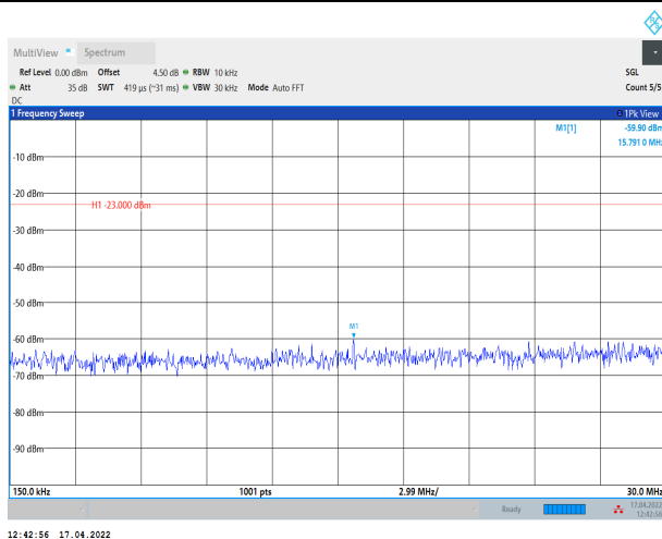
Band14-10MHz-QPSK-23330-1RB#0-Range2:0.15~30MHz
