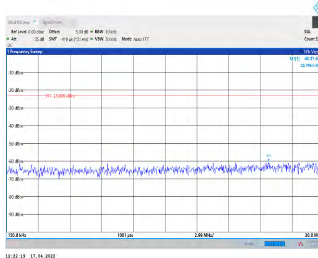
Band2-20MHz-QPSK-18700-1RB#0-Range2:0.15~30MHz
