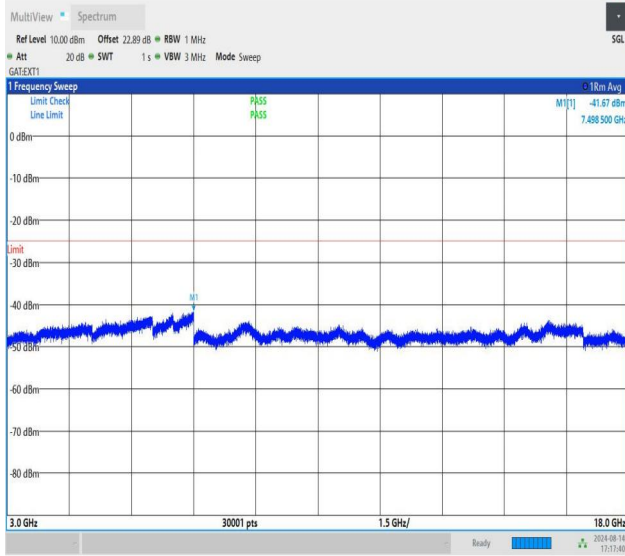
NTNV-n41-PC1.5-30-30-M-CP-QPSK-Edge_1RB_Left-3000-1800 0-PASS
