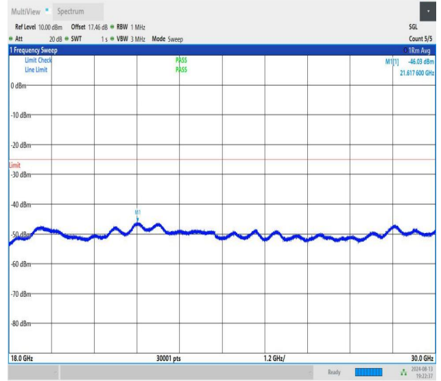
NTNV-n41-PC1.5-30-50-M-CP-QPSK-Edge_1RB_Left-18000-3000 0-PASS
