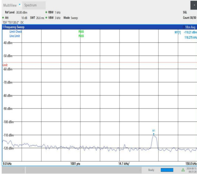
NTNV-n41-PC1.5-30-20-M-CP-QPSK-Edge_1RB_Left-0.009-0.15 -PASS
