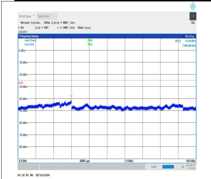
NTNV-n41-PC1.5-30-20-M-CP-QPSK-Edge_1RB_Left-3000-1800 0-PASS
