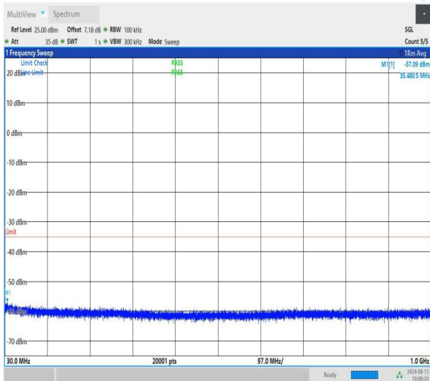
NTNV-n41-PC1.5-30-20-M-CP-QPSK-Edge_1RB_Left-30-1000-P ASS
