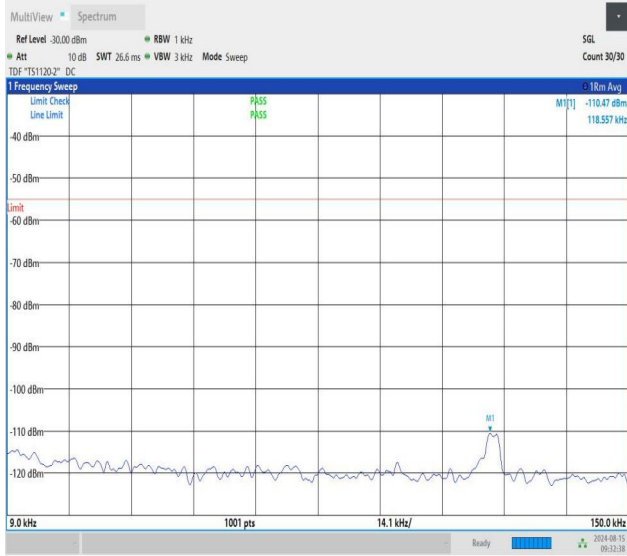
NTNV-n41-PC1.5-30-30-M-CP-QPSK-Edge_1RB_Left-0.009-0.15 -PASS
