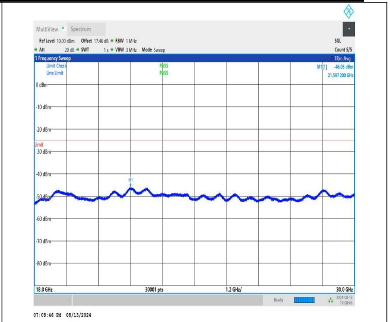
NTNV-n41-PC1.5-30-20-M-CP-QPSK-Edge_1RB_Left-18000-3000 0-PASS
