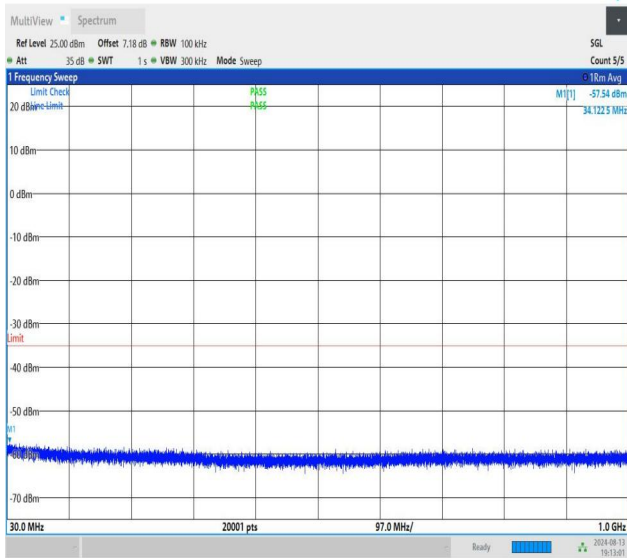
NTNV-n41-PC1.5-30-30-M-CP-QPSK-Edge_1RB_Left-30-1000-P ASS
