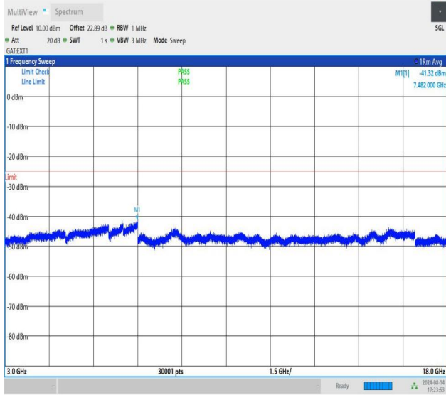
NTNV-n41-PC1.5-30-50-M-CP-QPSK-Edge_1RB_Left-3000-1800 0-PASS
