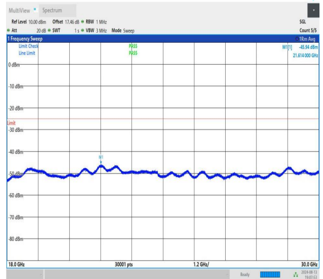
NTNV-n41-PC1.5-30-20-L-CP-QPSK-Edge_1RB_Right-18000-300 00-PASS
