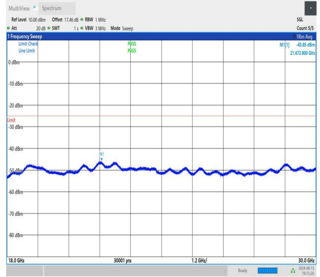
NTNV-n41-PC1.5-30-30-M-CP-QPSK-Edge_1RB_Left-18000-3000 0-PASS
