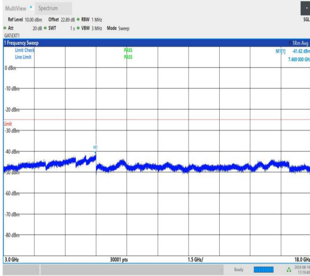
NTNV-n41-PC1.5-30-40-L-CP-QPSK-Edge_1RB_Left-3000-18000 -PASS
