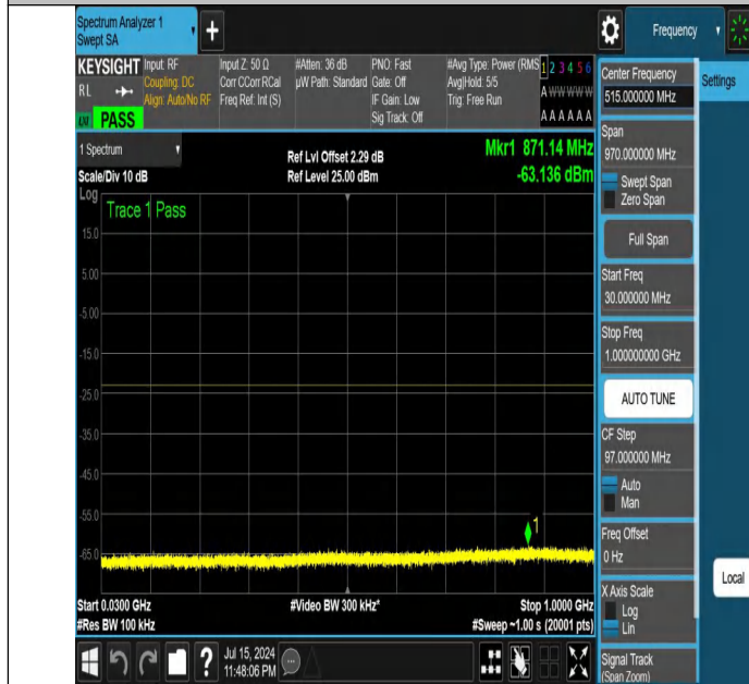
NTNV-DC_12A_n25A-PC3-15-5+20-M+L-N/A-N/A-DFT-PI2BPSK- Edge_1RB_Left-30-1000-PASS
