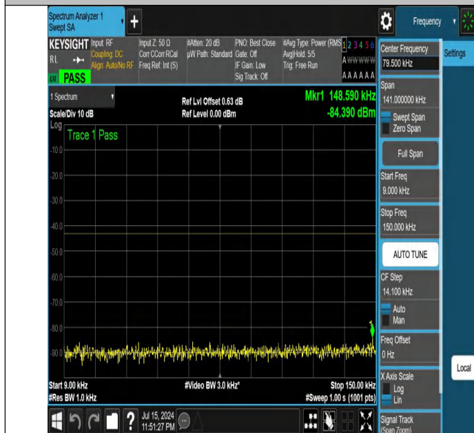
NTNV-DC_12A_n25A-PC3-15-5+20-M+L-N/A-N/A-DFT-QPSK-Edge e_1RB_Right-0.009-0.15-PASS
