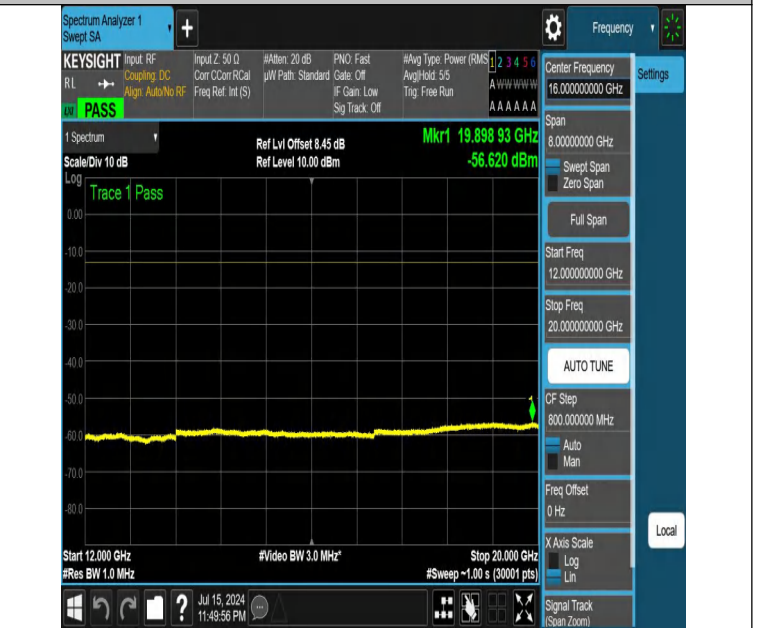
NTNV-DC_12A_n25A-PC3-15-5+20-M+L-N/A-N/A-DFT-PI2BPSK-E dge_1RB_Right-12000-20000-PASS
