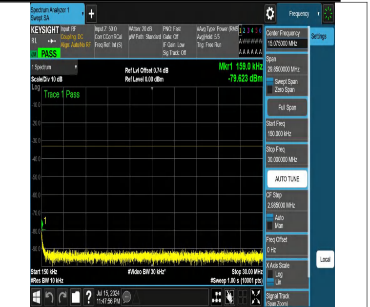
NTNV-DC_12A_n25A-PC3-15-5+20-M+L-N/A-N/A-DFT-PI2BPSK-E dge_1RB_Left-0.15-30-PASS
