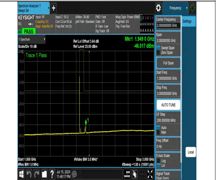
NTNV-DC_12A_n25A-PC3-15-5+20-M+L-N/A-N/A-DFT-PI2BPSK-E dge_1RB_Left-1000-3000-PASS
