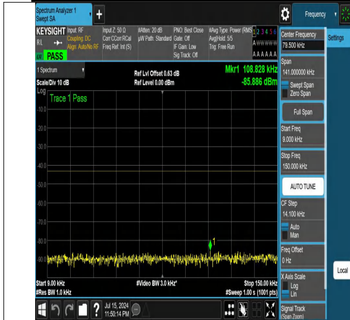
NTNV-DC_12A_n25A-PC3-15-5+20-M+L-N/A-N/A-DFT-QPSK-Edge e_1RB_Left-0.009-0.15-PASS
