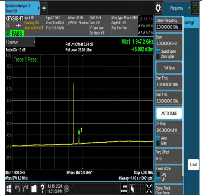
NTNV-DC_12A_n25A-PC3-15-5+20-M+L-N/A-N/A-DFT-QPSK-Edge _1RB_Right-1000-3000-PASS
