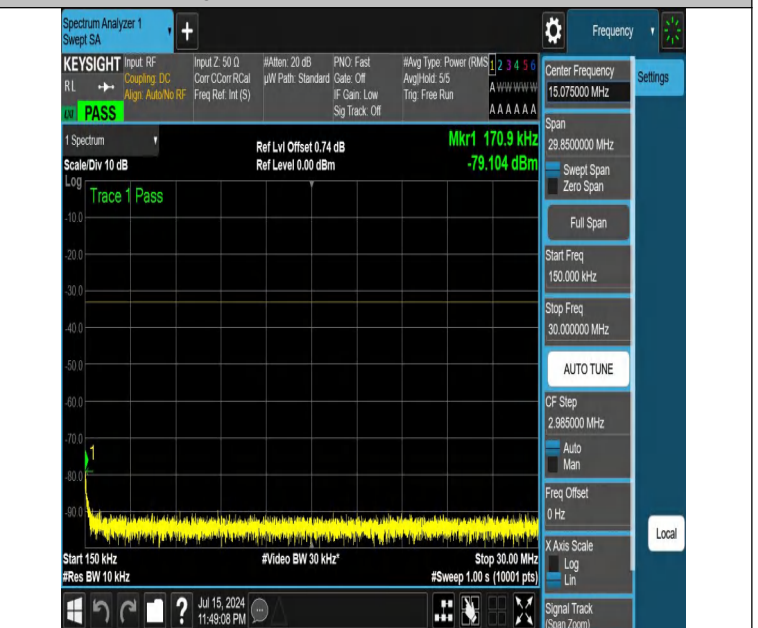
NTNV-DC_12A_n25A-PC3-15-5+20-M+L-N/A-N/A-DFT-PI2BPSK-E dge_1RB_Right-0.15-30-PASS
