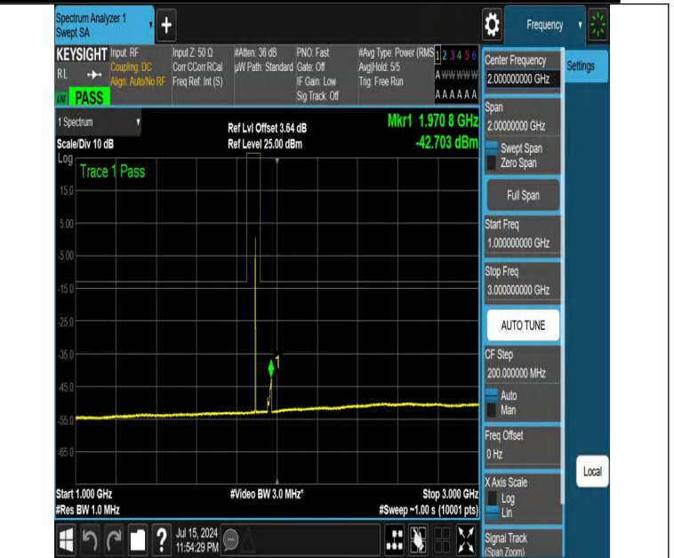
NTNV-DC_12A_n25A-PC3-15-5+20-M+M-N/A-N/A-DFT-PI2BPSK-E dge_1RB_Right-1000-3000-PASS
