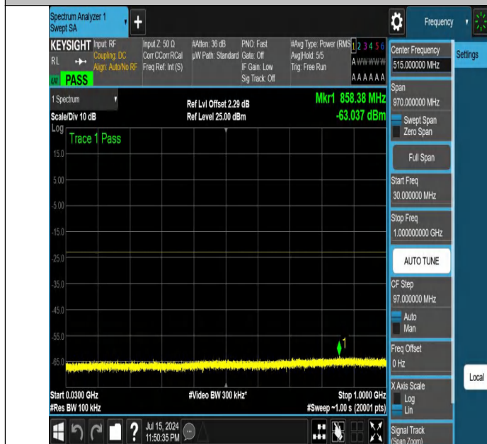
NTNV-DC_12A_n25A-PC3-15-5+20-M+L-N/A-N/A-DFT-QPSK-Edge e_1RB_Left-30-1000-PASS
