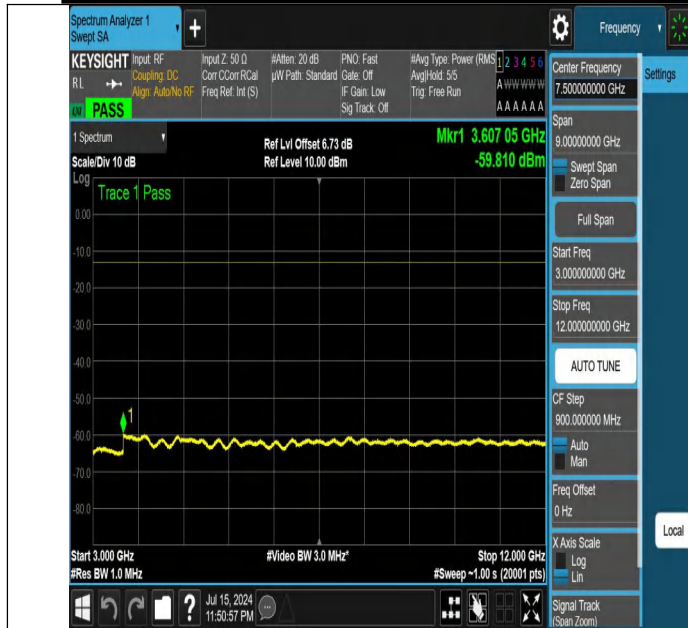
NTNV-DC_12A_n25A-PC3-15-5+20-M+L-N/A-N/A-DFT-QPSK-Edge e_1RB_Left-3000-12000-PASS
