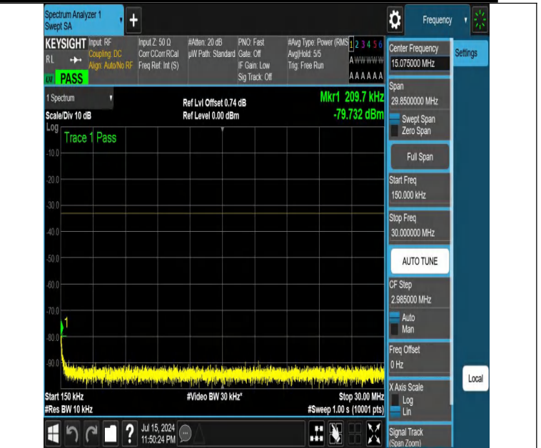
NTNV-DC_12A_n25A-PC3-15-5+20-M+L-N/A-N/A-DFT-QPSK-Edge _1RB_Left-0.15-30-PASS
