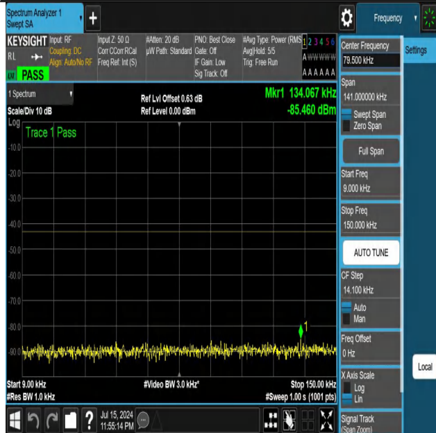
NTNV-DC_12A_n25A-PC3-15-5+20-M+M-N/A-N/A-DFT-QPSK-Edge_1RB_Left-0.009-0.15-PASS
