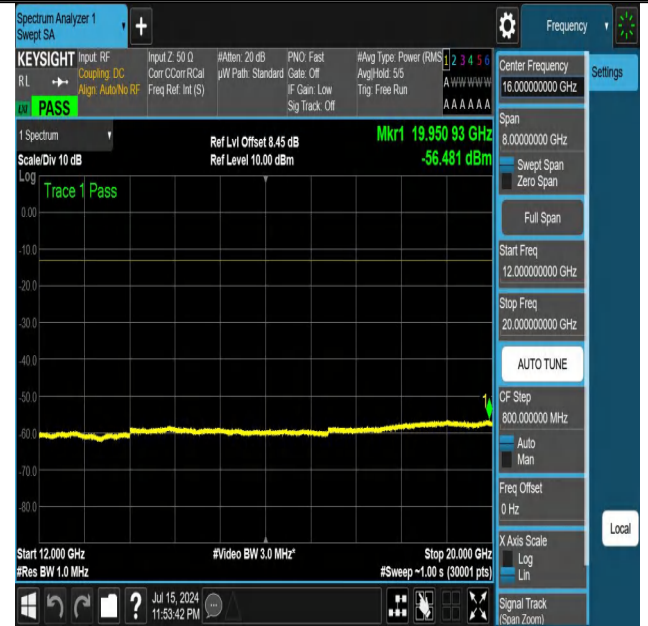
NTNV-DC_12A_n25A-PC3-15-5+20-M+M-N/A-N/A-DFT-PI2BPSK-E dge_1RB_Left-12000-20000-PASS
