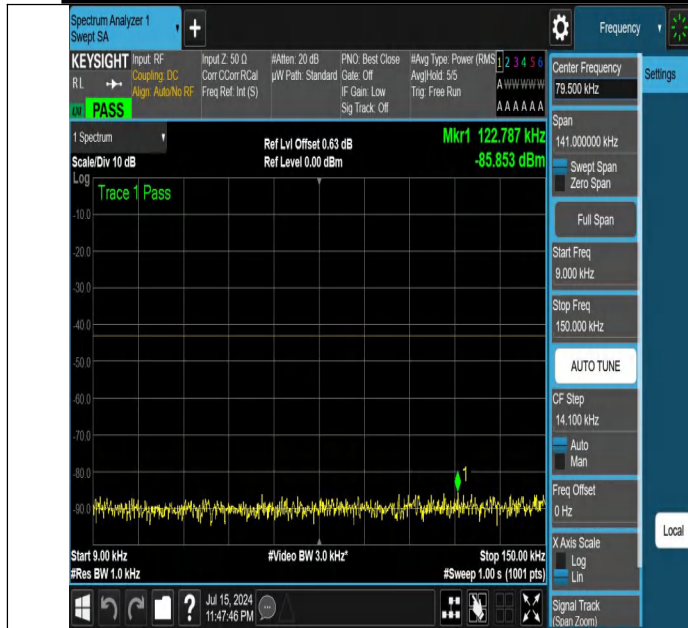
NTNV-DC_12A_n25A-PC3-15-5+20-M+L-N/A-N/A-DFT-PI2BPSK- Edge_1RB_Left-0.009-0.15-PASS
