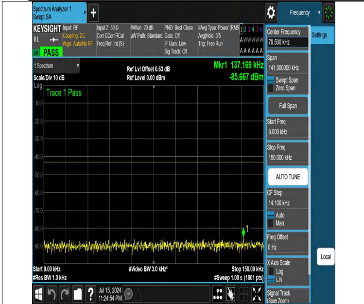
NTNV-DC_12A_n25A-PC3-15-5+10-M+M-N/A-N/A-DFT-QPSK-Edge_1RB_Left-0.009-0.15-PASS
