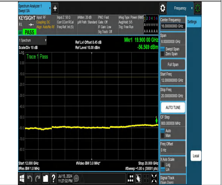
NTNV-DC_12A_n25A-PC3-15-5+10-M+M-N/A-N/A-DFT-QPSK-Edge_1RB_Right-12000-20000-PASS
