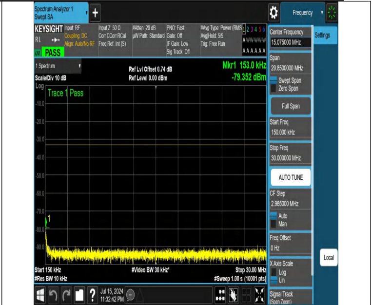
NTNV-DC_12A_n25A-PC3-15-5+15-M+L-N/A-N/A-DFT-PI2BPSK-E dge_1RB_Left-0.15-30-PASS
