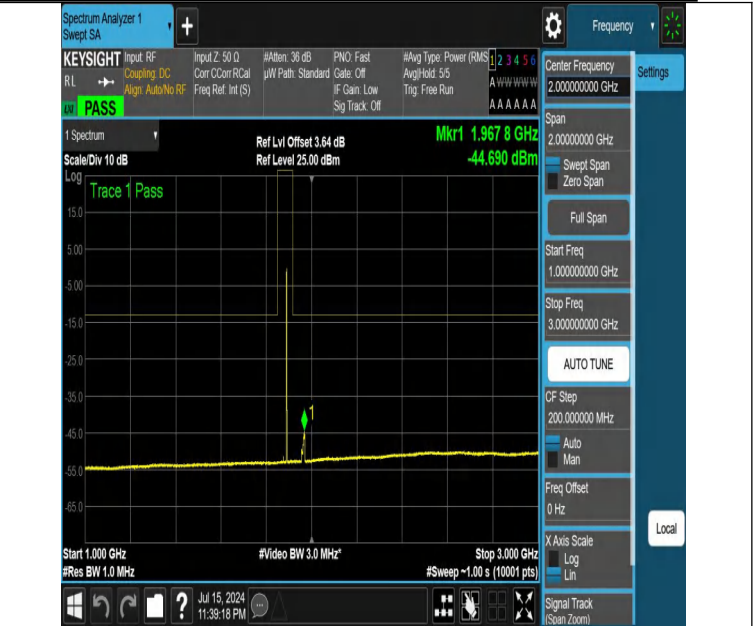
NTNV-DC_12A_n25A-PC3-15-5+15-M+M-N/A-N/A-DFT-PI2BPSK-E dge_1RB_Right-1000-3000-PASS
