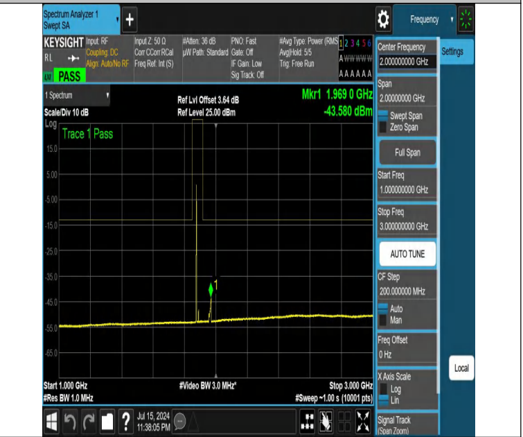
NTNV-DC_12A_n25A-PC3-15-5+15-M+M-N/A-N/A-DFT-PI2BPSK-E dge_1RB_Left-1000-3000-PASS
