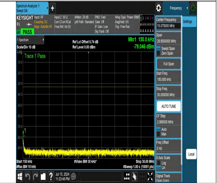
NTNV-DC_12A_n25A-PC3-15-5+10-M+M-N/A-N/A-DFT-PI2BPSK-E dge_1RB_Right-0.15-30-PASS
