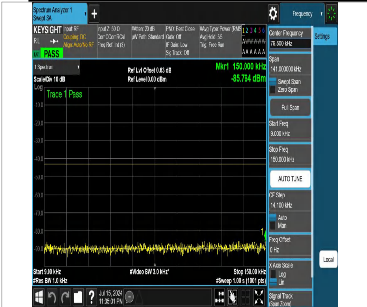
NTNV-DC_12A_n25A-PC3-15-5+15-M+L-N/A-N/A-DFT-QPSK-Edge e_1RB_Left-0.009-0.15-PASS
