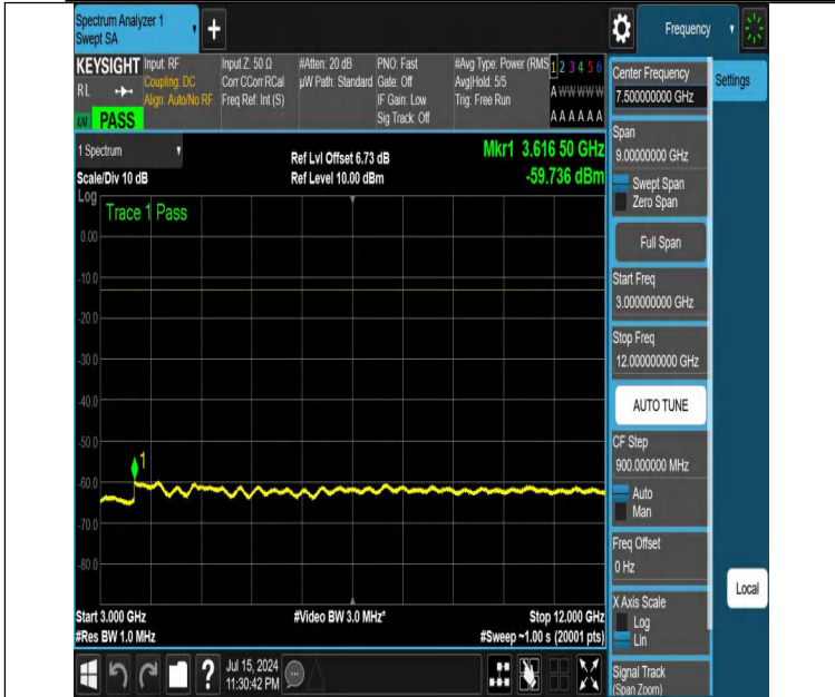
NTNV-DC_12A_n25A-PC3-15-5+10-M+H-N/A-N/A-DFT-QPSK-Edge e_1RB_Left-3000-12000-PASS
