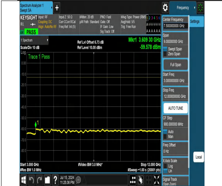
NTNV-DC_12A_n25A-PC3-15-5+10-M+M-N/A-N/A-DFT-QPSK-Edge_1RB_Left-3000-12000-PASS
