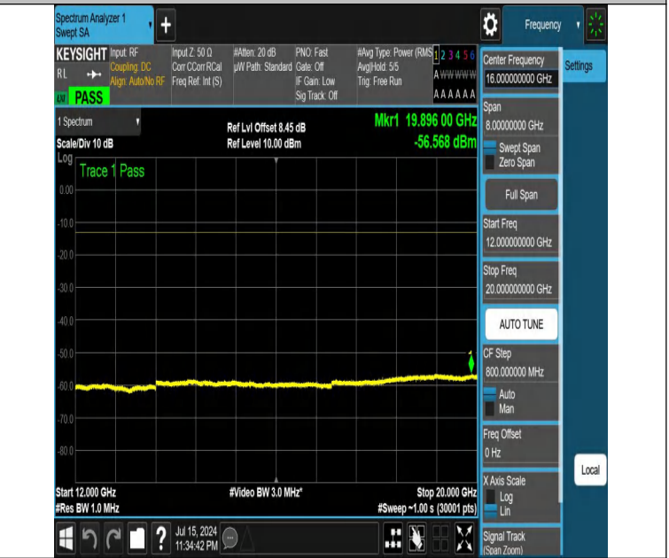
NTNV-DC_12A_n25A-PC3-15-5+15-M+L-N/A-N/A-DFT-PI2BPSK-E dge_1RB_Right-12000-20000-PASS
