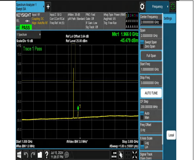
NTNV-DC_12A_n25A-PC3-15-5+10-M+M-N/A-N/A-DFT-QPSK-Edge_1RB_Right-1000-3000-PASS
