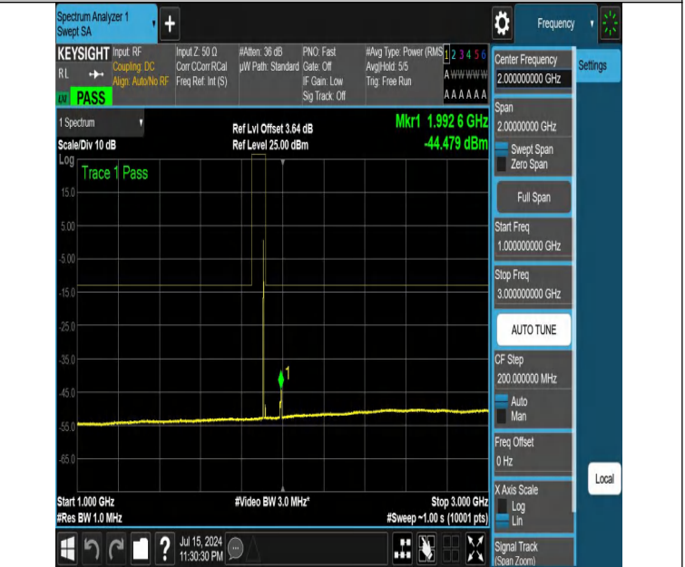
NTNV-DC_12A_n25A-PC3-15-5+10-M+H-N/A-N/A-DFT-QPSK-Edg e_1RB_Left-1000-3000-PASS
