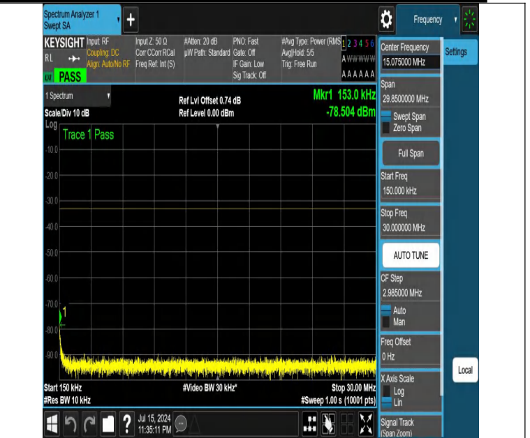
NTNV-DC_12A_n25A-PC3-15-5+15-M+L-N/A-N/A-DFT-QPSK-Edge _1RB_Left-0.15-30-PASS
