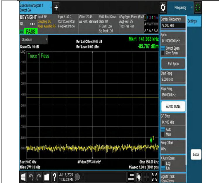
NTNV-DC_12A_n25A-PC3-15-5+15-M+L-N/A-N/A-DFT-PI2BPSK-Edge_1RB_Left-0.009-0.15-PASS
