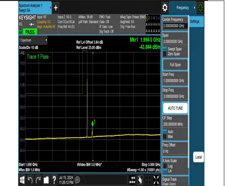
NTNV-DC_12A_n25A-PC3-15-5+10-M+H-N/A-N/A-DFT-PI2BPSK-E dge_1RB_Right-1000-3000-PASS
