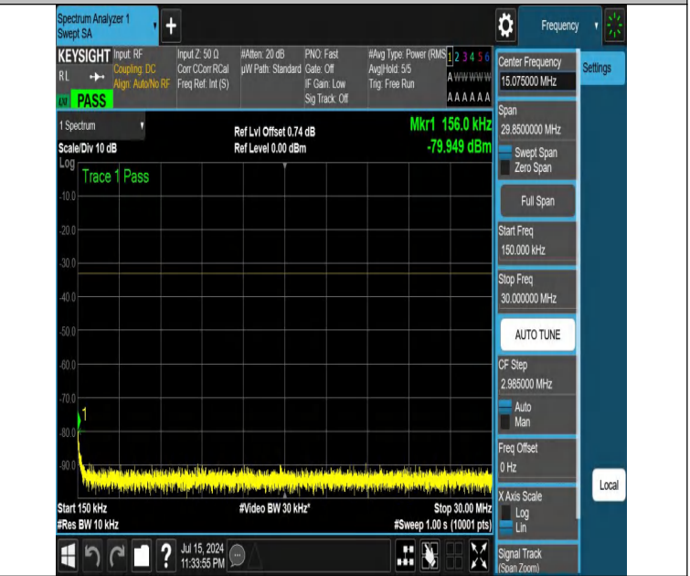
NTNV-DC_12A_n25A-PC3-15-5+15-M+L-N/A-N/A-DFT-PI2BPSK-E dge_1RB_Right-0.15-30-PASS
