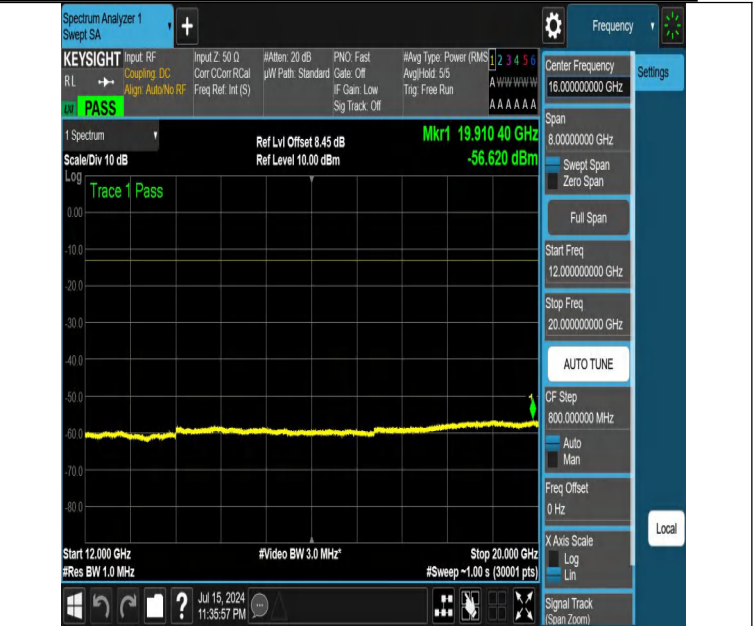
NTNV-DC_12A_n25A-PC3-15-5+15-M+L-N/A-N/A-DFT-QPSK-Edge _1RB_Left-12000-20000-PASS
