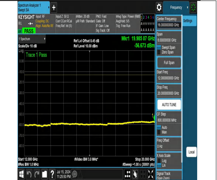
NTNV-DC_12A_n25A-PC3-15-5+10-M+M-N/A-N/A-DFT-QPSK-Edge_1RB_Left-12000-20000-PASS
