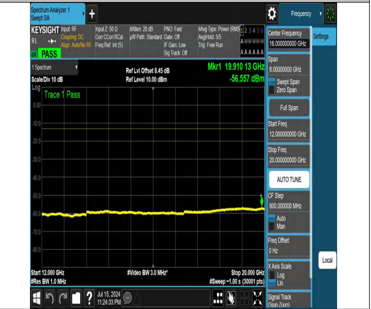
NTNV-DC_12A_n25A-PC3-15-5+10-M+M-N/A-N/A-DFT-PI2BPSK-E dge_1RB_Right-12000-20000-PASS
