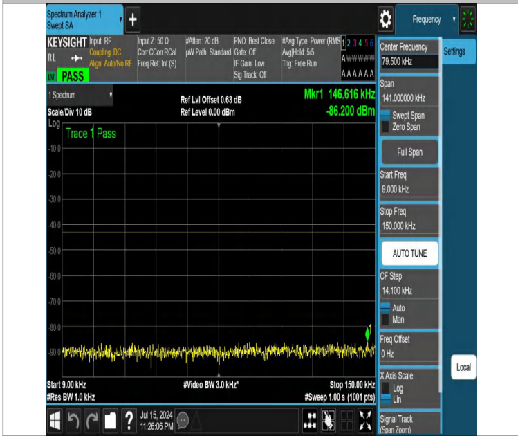
NTNV-DC_12A_n25A-PC3-15-5+10-M+M-N/A-N/A-DFT-QPSK-Edge_1RB_Right-0.009-0.15-PASS
