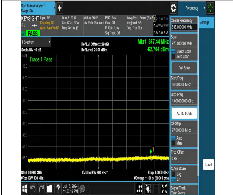
NTNV-DC_12A_n25A-PC3-15-5+10-M+H-N/A-N/A-DFT-QPSK-Edg e_1RB_Left-30-1000-PASS
