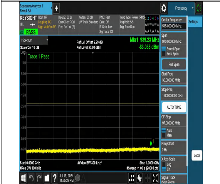
NTNV-DC_12A_n25A-PC3-15-5+15-M+L-N/A-N/A-DFT-QPSK-Edge e_1RB_Left-30-1000-PASS
