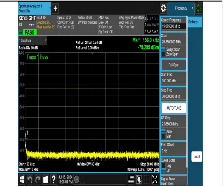
NTNV-DC_12A_n25A-PC3-15-5+10-M+H-N/A-N/A-DFT-PI2BPSK-E dge_1RB_Right-0.15-30-PASS
