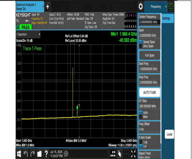
NTNV-DC_12A_n25A-PC3-15-5+10-M+M-N/A-N/A-DFT-PI2BPSK-E dge_1RB_Right-1000-3000-PASS
