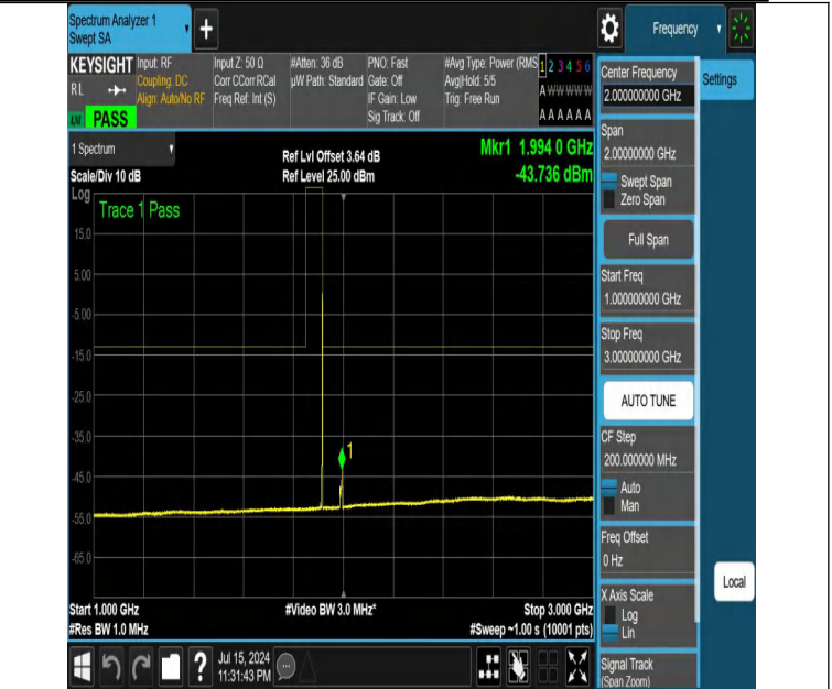
NTNV-DC_12A_n25A-PC3-15-5+10-M+H-N/A-N/A-DFT-QPSK-Edge e_1RB_Right-1000-3000-PASS
