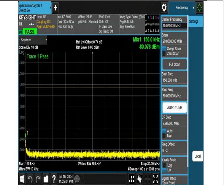
NTNV-DC_12A_n25A-PC3-15-5+10-M+M-N/A-N/A-DFT-QPSK-Edge_1RB_Left-0.15-30-PASS
