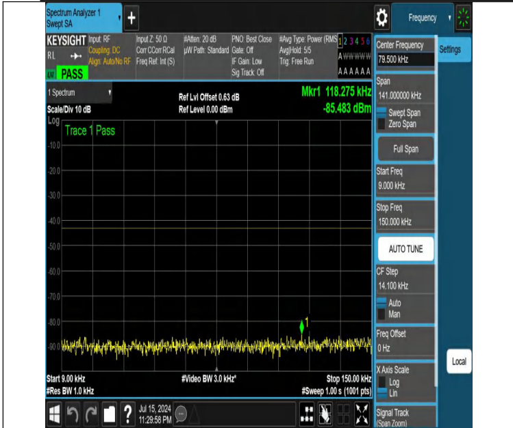
NTNV-DC_12A_n25A-PC3-15-5+10-M+H-N/A-N/A-DFT-QPSK-Edg e_1RB_Left-0.009-0.15-PASS
