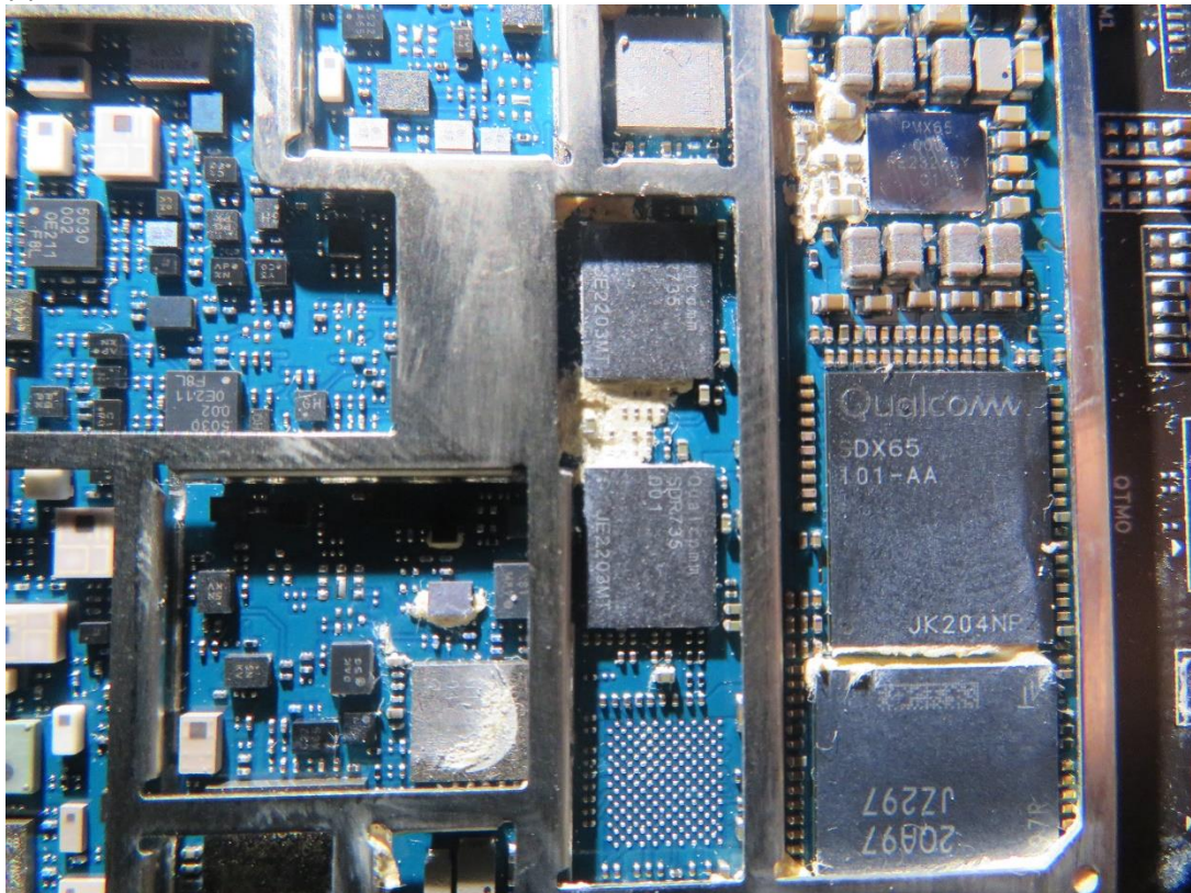
(3) EUT Photo
