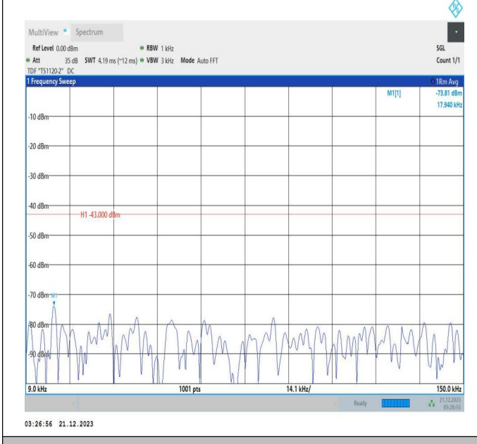
66-66-5MHz-20MHz-QPSK-QPSK-132428-132572-1RB#0-1 RB#99-0.009~0.15MHz-PASS
