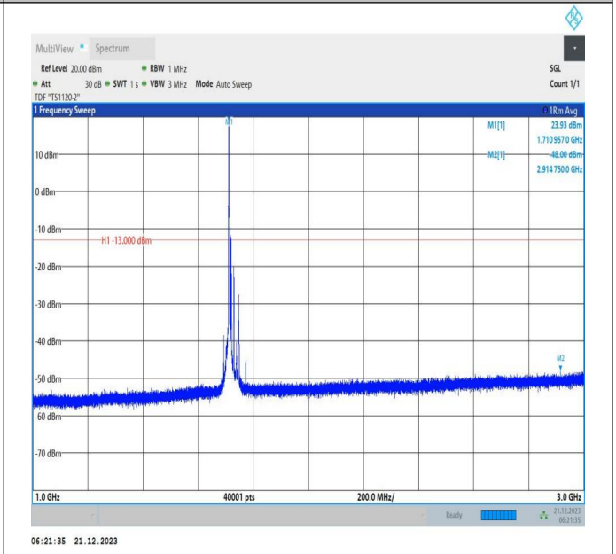
66-66-10MHz-15MHz-QPSK-QPSK-132025-132145-1RB#0-ORB#0-1000~3000MHz-PASS
