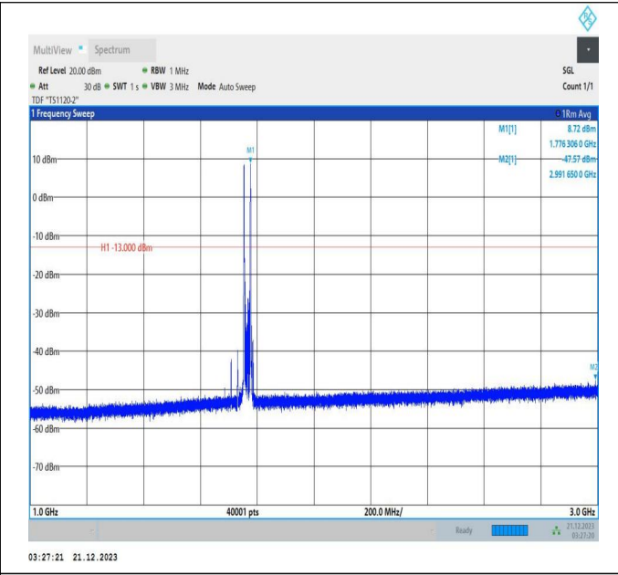
66-66-5MHz-20MHz-QPSK-QPSK-132428-132572-1RB#0-1 RB#99-1000~3000MHz-PASS
