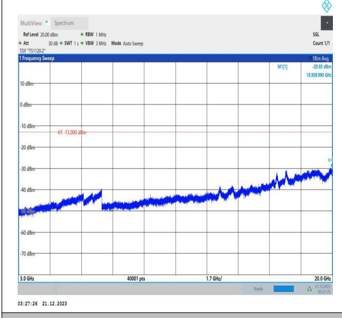
66-66-5MHz-20MHz-QPSK-QPSK-132428-132572-1RB#0-1 RB#99-3000~20000MHz-PASS
