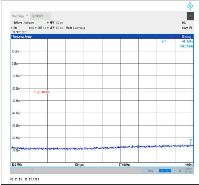
66-66-5MHz-20MHz-QPSK-QPSK-132428-132572-1RB#0-1 RB#99-30~1000MHz-PASS
