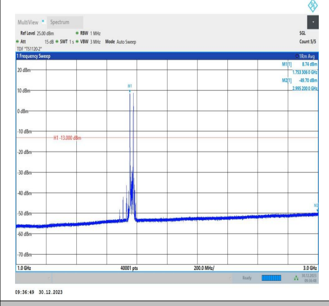
66-66-5MHz-20MHz-64QAM-64QAM-132428-132572-1RB#0 -1RB#99-1000~3000MHz-PASS
