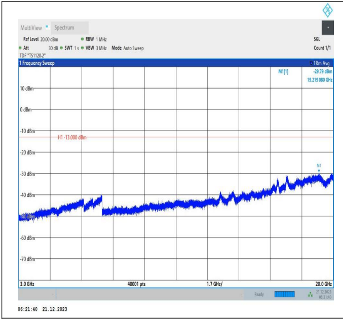
66-66-10MHz-15MHz-QPSK-QPSK-132025-132145-1RB#0-ORB#0-3000~20000MHz-PASS
