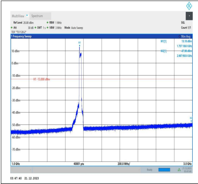
66-66-5MHz-20MHz-QPSK-QPSK-132428-132572-25RB#0-100RB#0-1000~3000MHz-PASS
