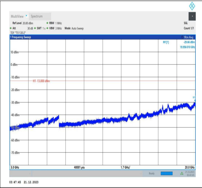
66-66-5MHz-20MHz-QPSK-QPSK-132428-132572-25RB#0-100RB#0-3000~20000MHz-PASS
