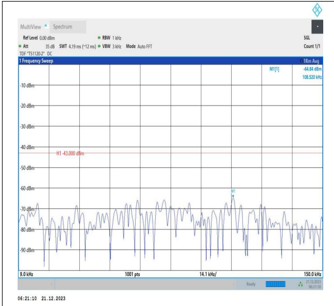
66-66-10MHz-15MHz-QPSK-QPSK-132025-132145-1RB#0-ORB#0-0.009~0.15MHz-PASS
