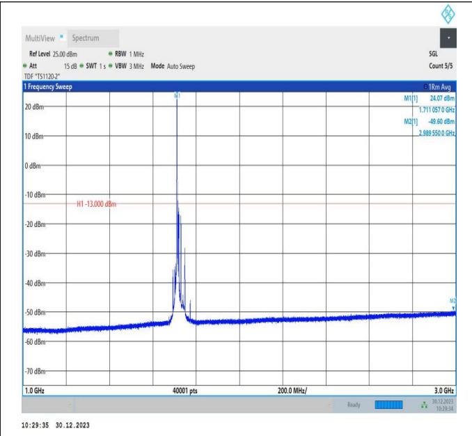
66-66-10MHz-15MHz-64QAM-64QAM-132025-132145-1RB# 0-ORB#0-1000~3000MHz-PASS
