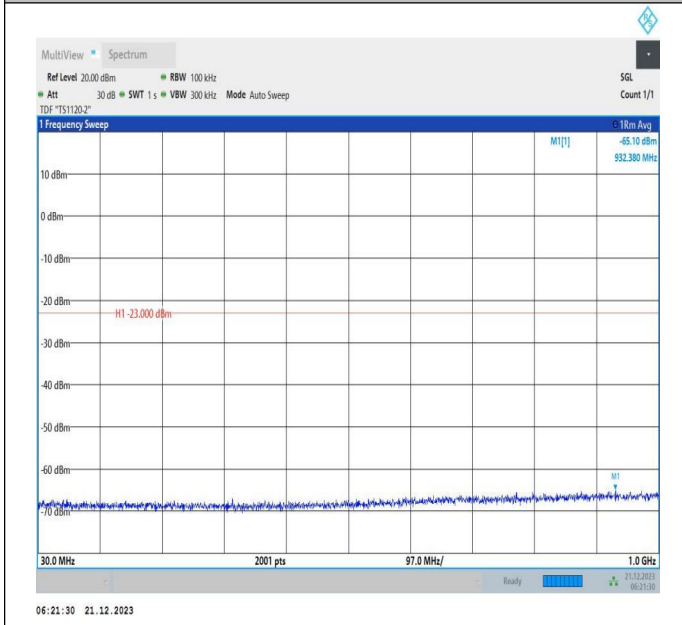
66-66-10MHz-15MHz-QPSK-QPSK-132025-132145-1RB#0-ORB#0-30~1000MHz-PASS
