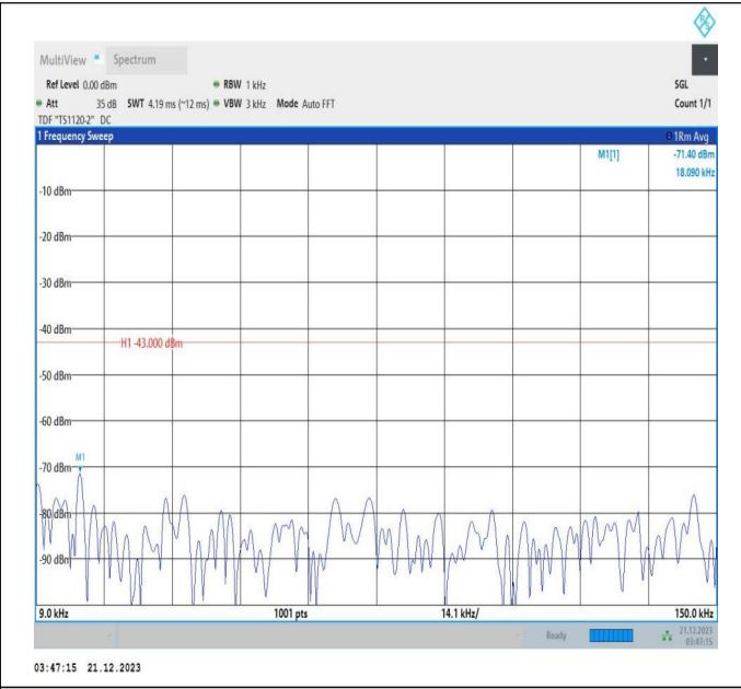
66-66-5MHz-20MHz-QPSK-QPSK-132428-132572-25RB#0-100RB#0-0.009~0.15MHz-PASS
