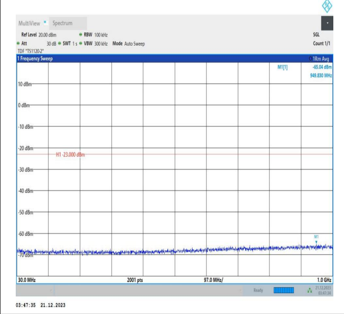
66-66-5MHz-20MHz-QPSK-QPSK-132428-132572-25RB#0-100RB#0-30~1000MHz-PASS
